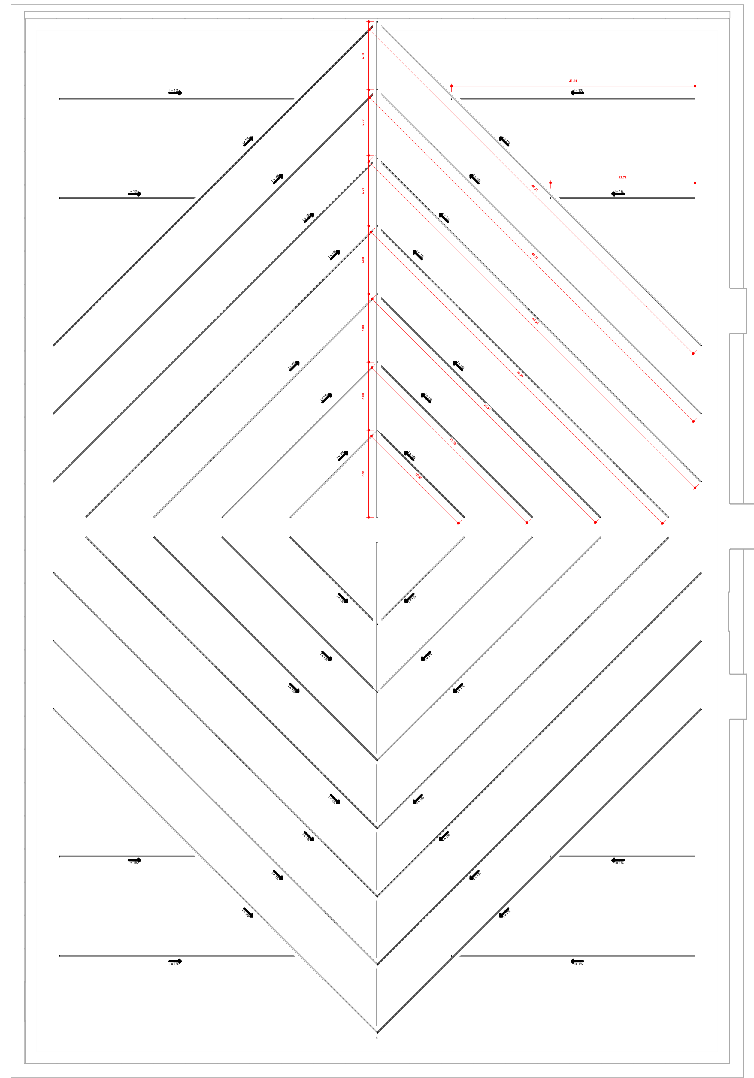
3 Drenagem Escala: 1 : 200
