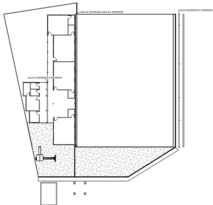
② Nível 1 ÁGUAS PLUVIAIS 1 : 200
