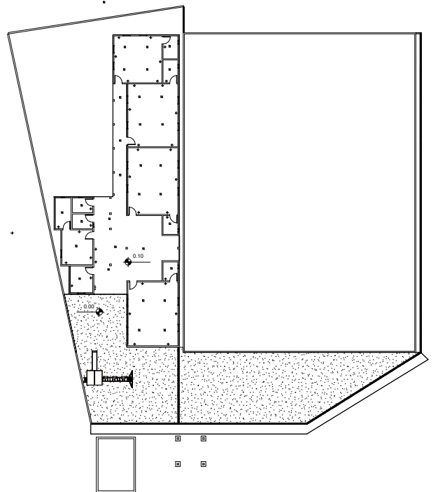
① Nível 1 elétrico 1 : 200
