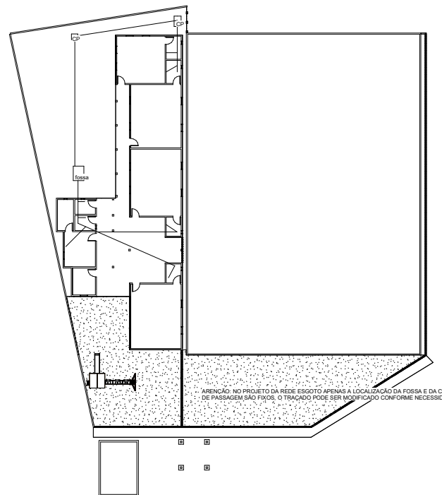
② Nível 1 esgoto 1 : 200
