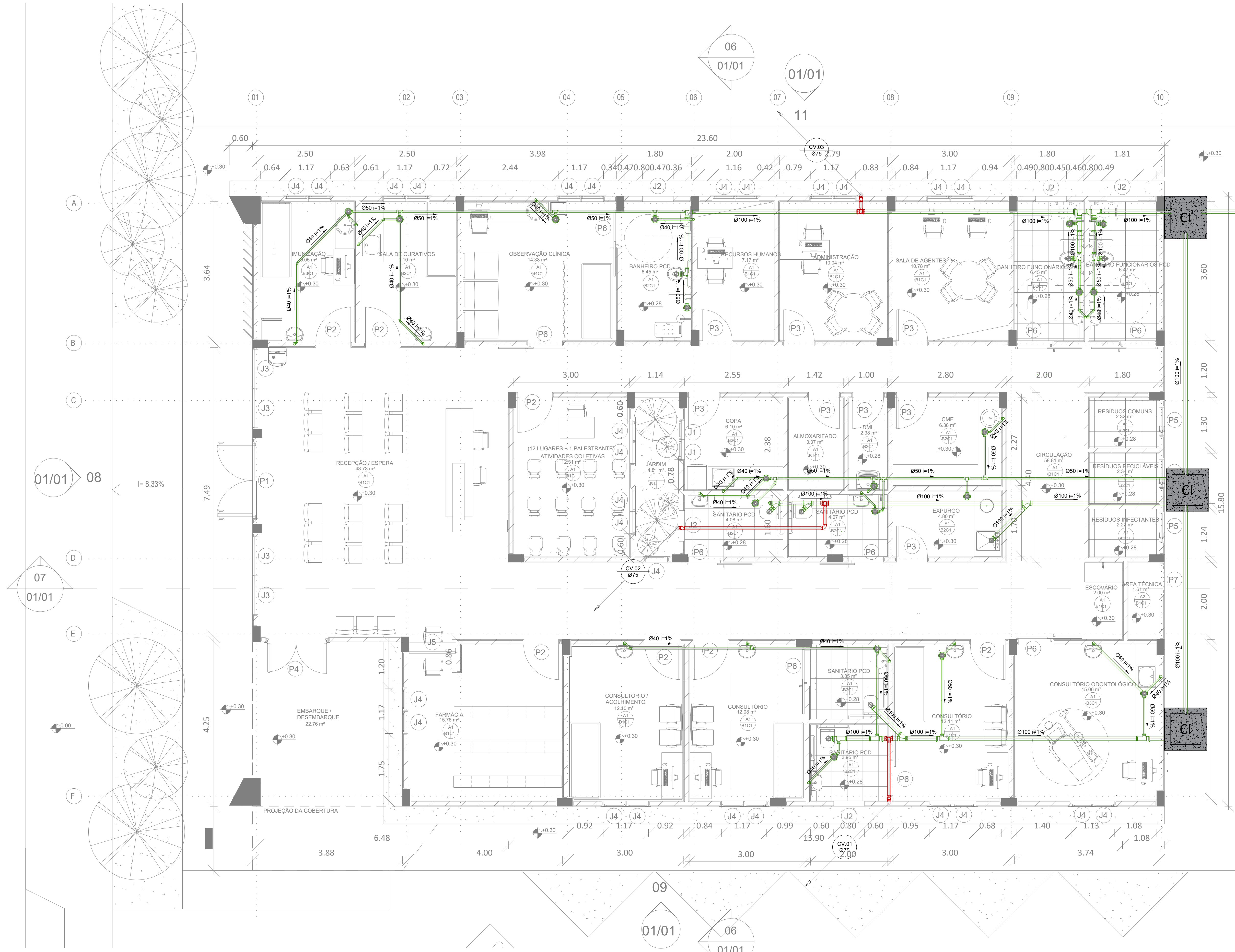
32 PLANTA BAIXA TÉRREO 1:100
