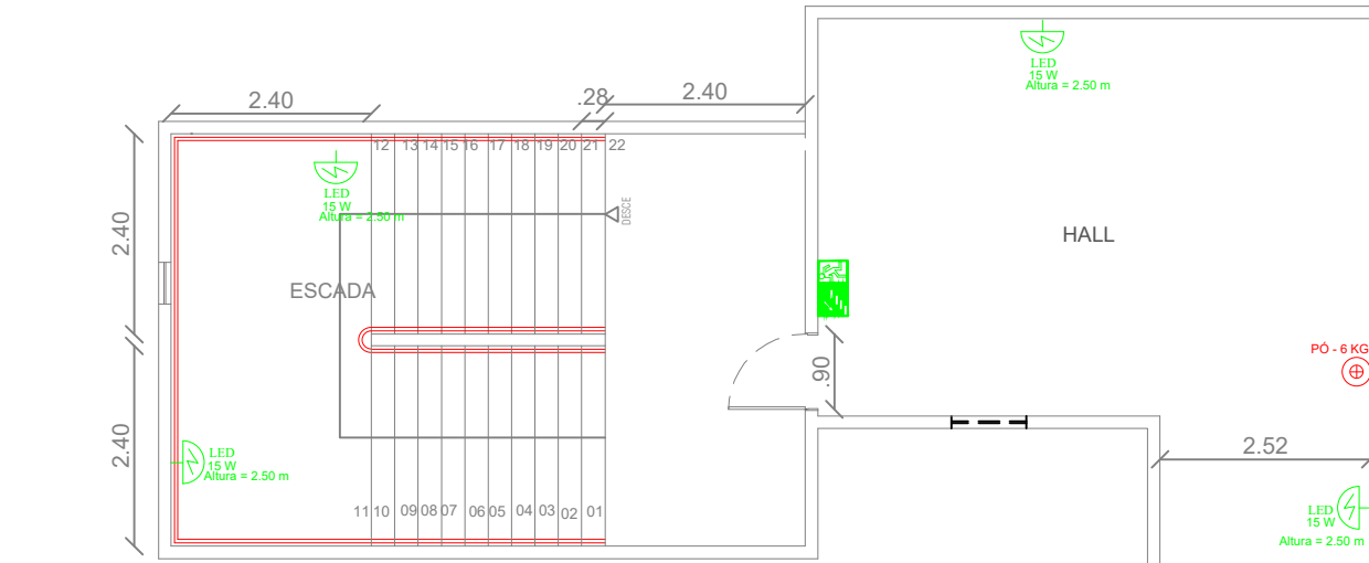
2 Planta Baixa - 1º Pav.
