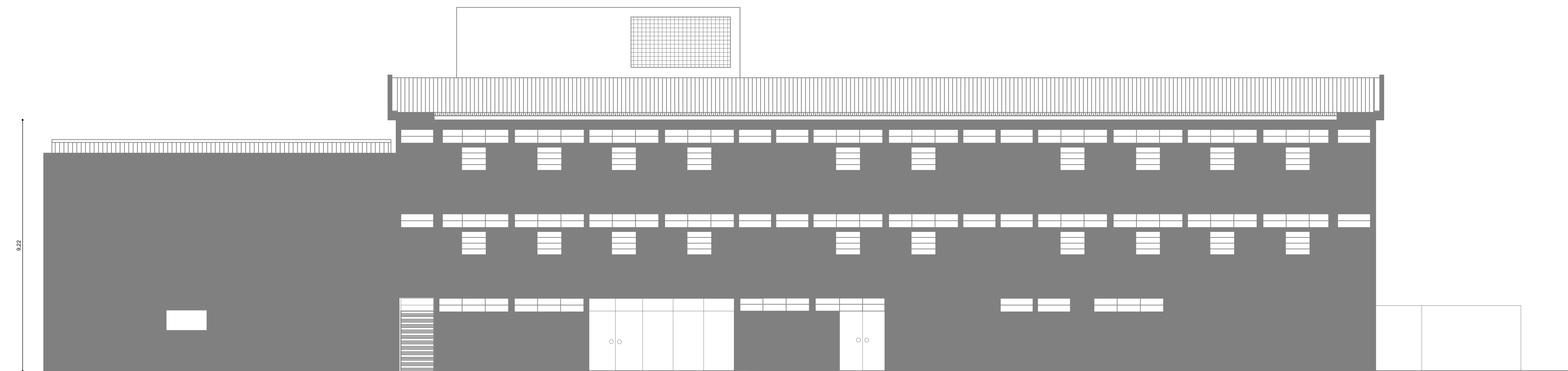
3 Fachada ESCALA 1:100
