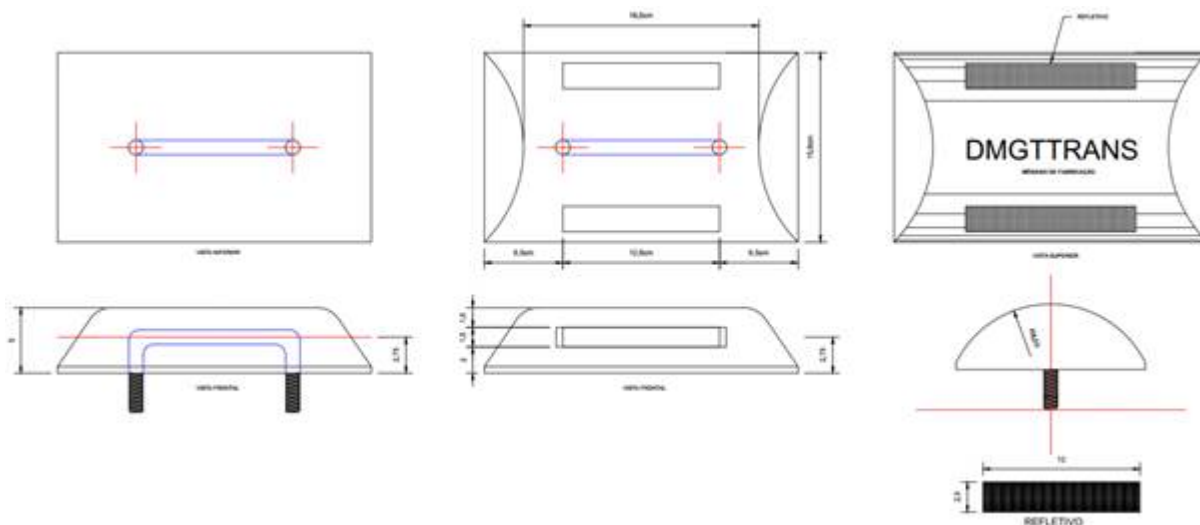
Figura 1 - Tachão refletivo
