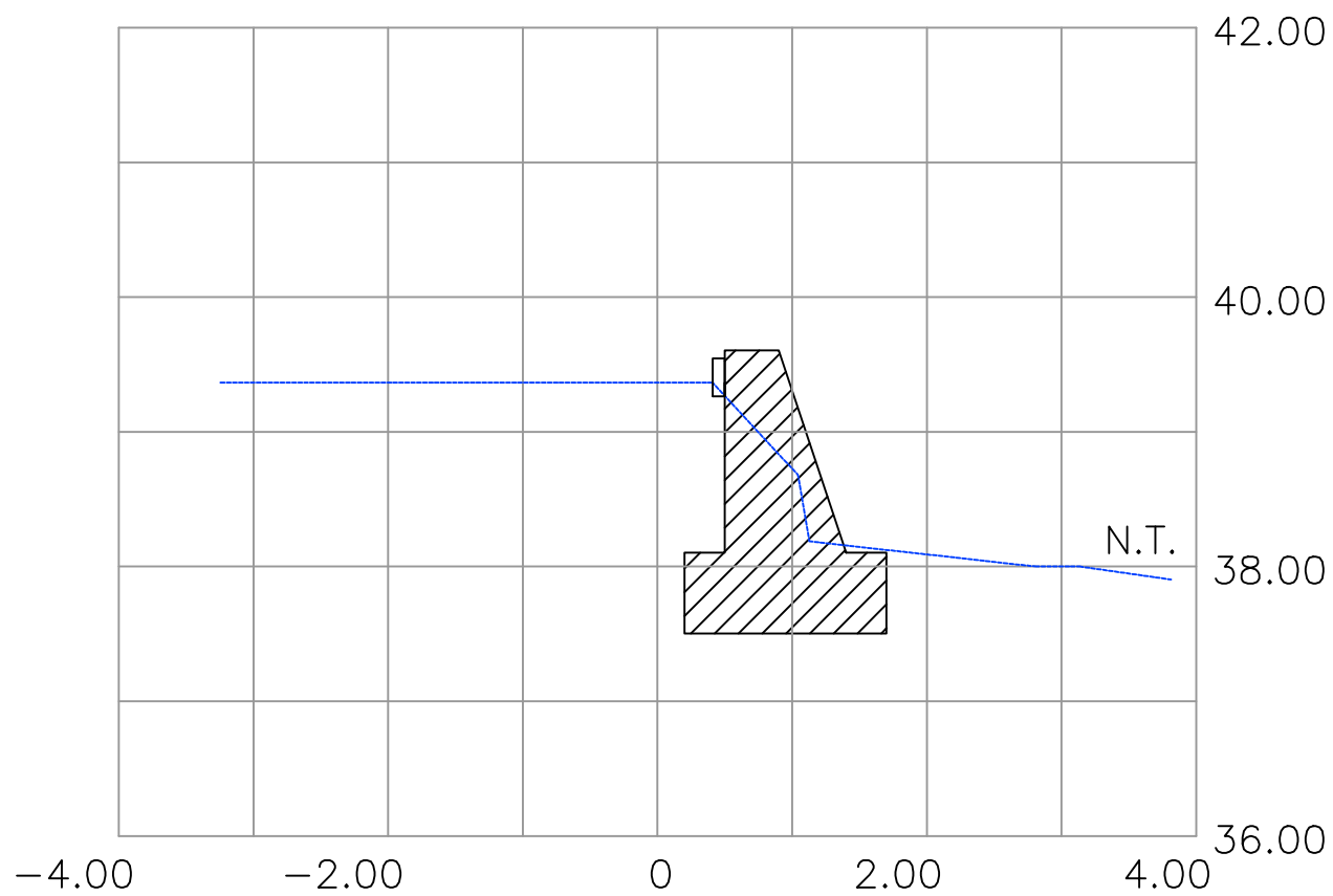
PERFIL GEOMÉTRICO - MURO - RUA MANOEL FERREIRA DA COSTA
