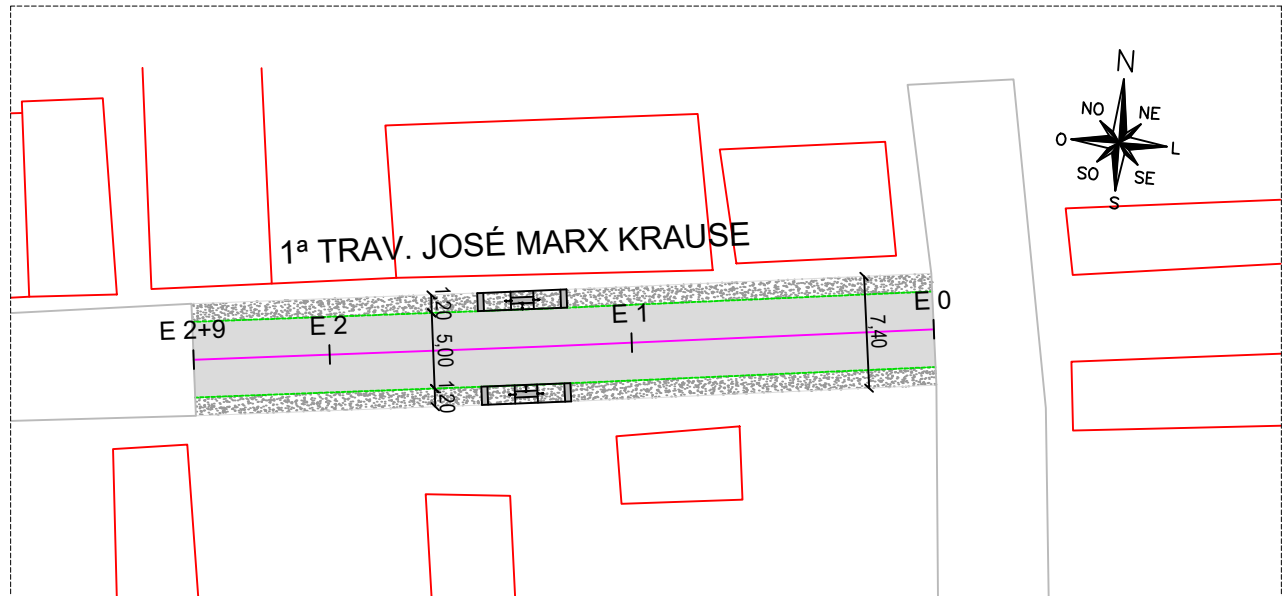
GEOMÉTRICO Escala 1/500
