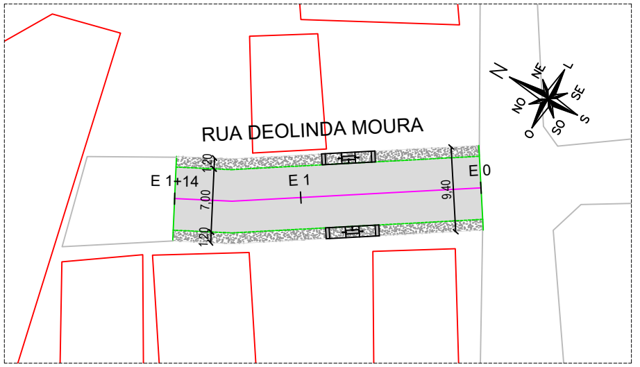
GEOMÉTRICO Escala 1/500
