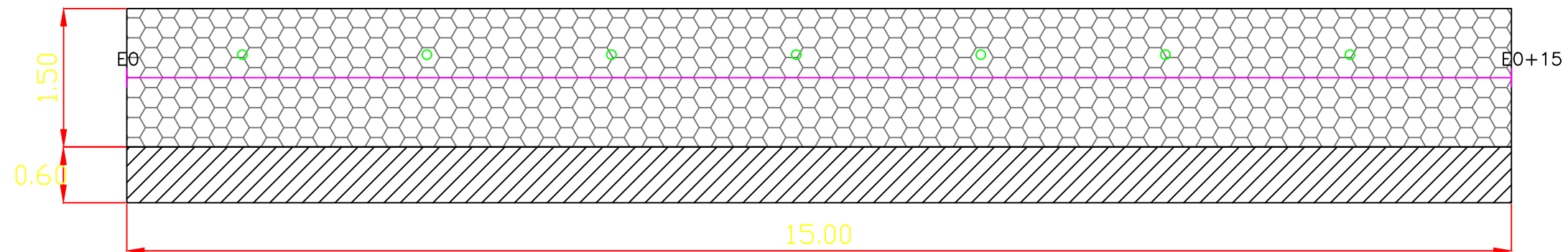
PLANTA GEOMÉTRICA - MURO - RUA MANOEL FERREIRA DA COSTA
