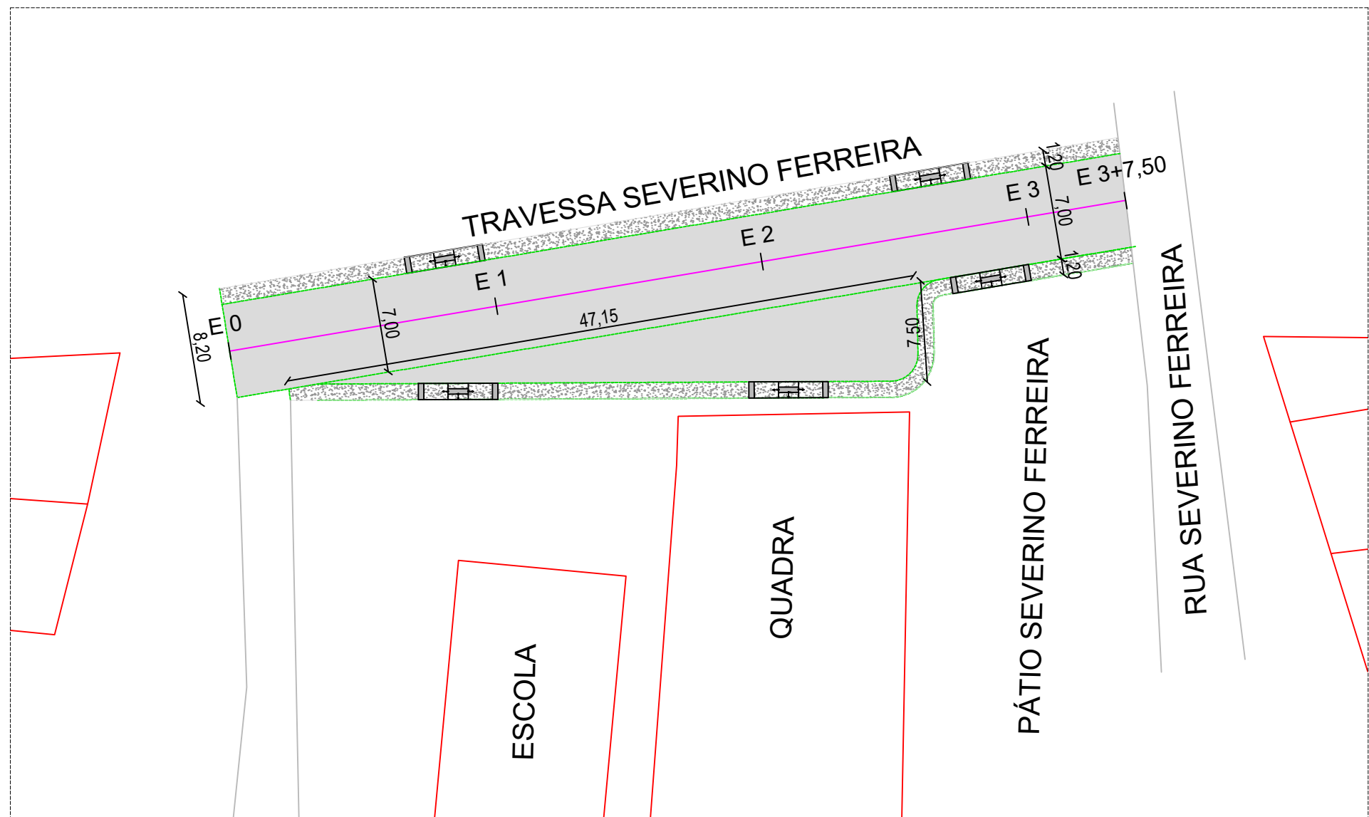
GEOMÉTRICO Escala 1/500
