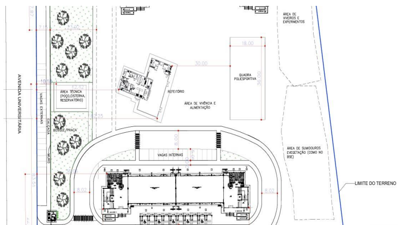
Figura 1: Planta de Locação Restaurante Universitário e Quadra de Esportes do Campus Rurópolis
