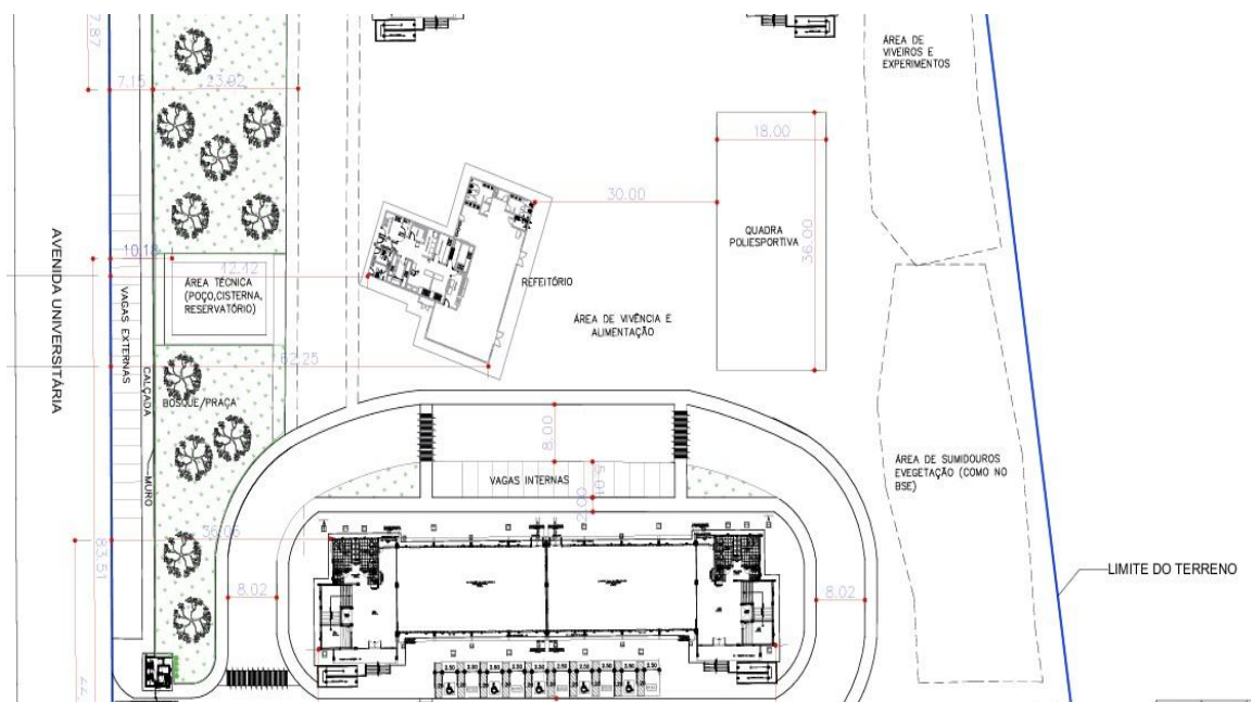
Figura 5: Planta de Localização Restaurante Universitário e Quadra de Esportes do Campus Rurópolis
