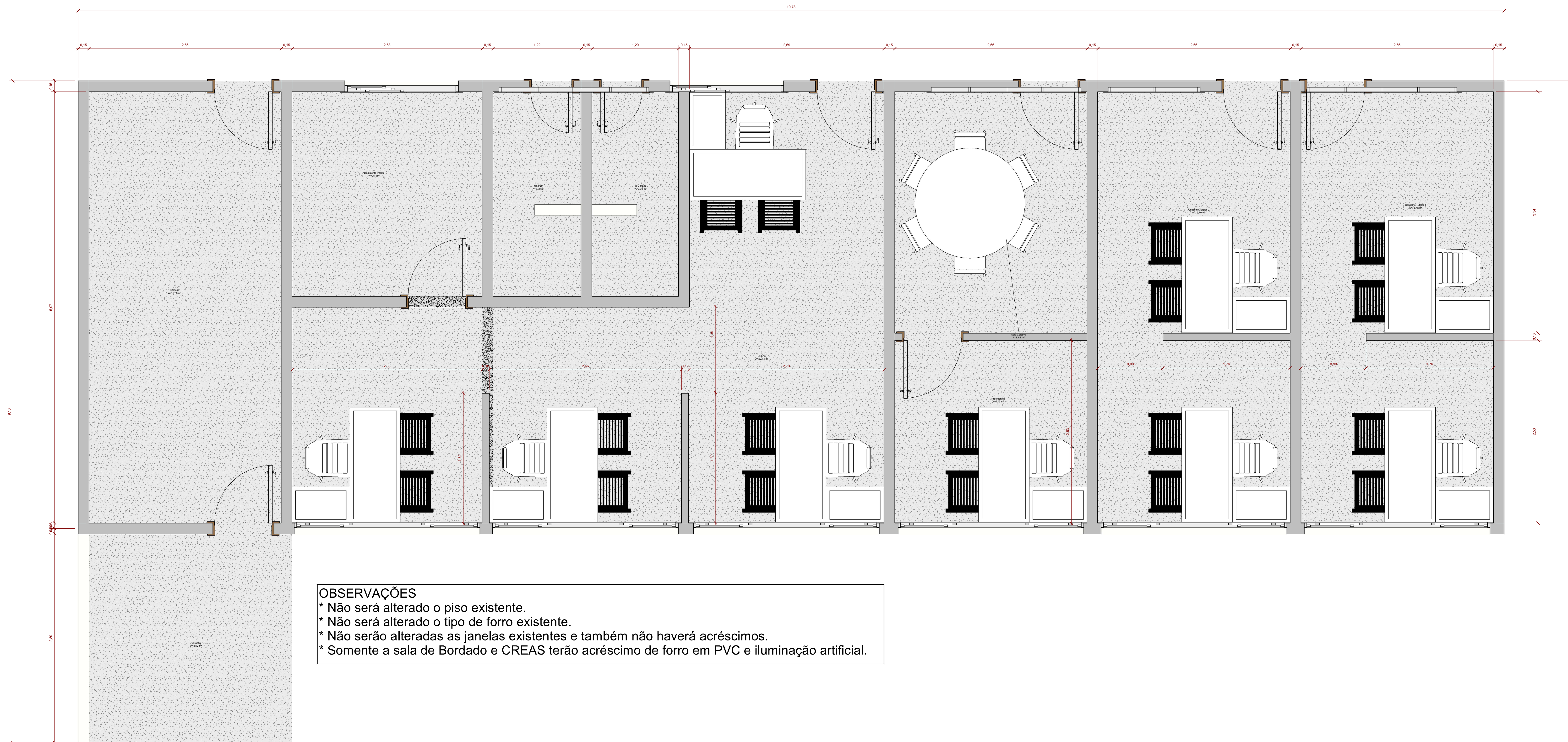
Planta Baixa - 1 CREAS/Conselho 1:25
