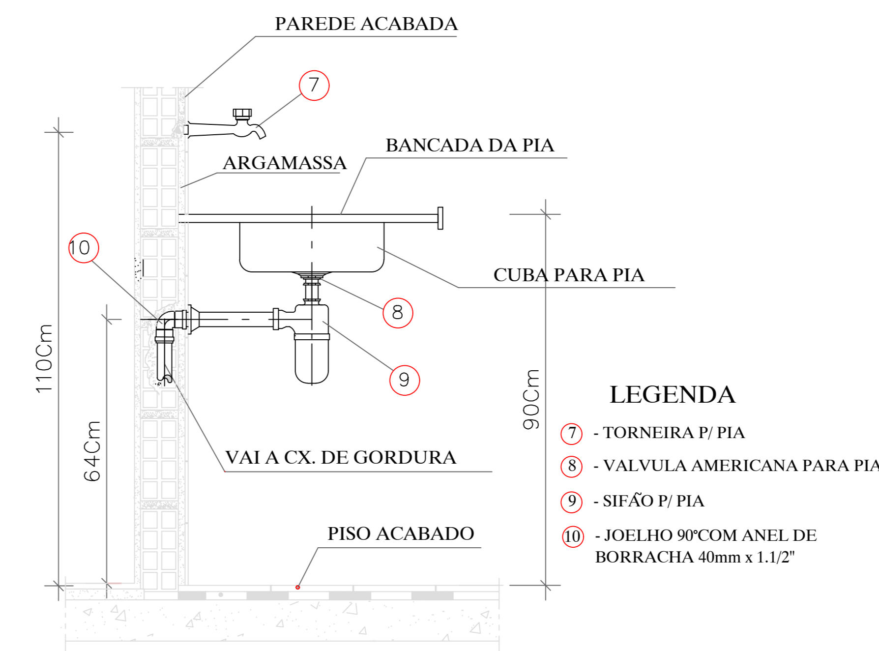
DET. LIGAÇÃO DA PIA S/ ESCALA
