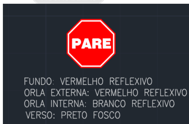
Figura 2. Placa R1 – parada obrigatória, com lado de 0,248 m.
