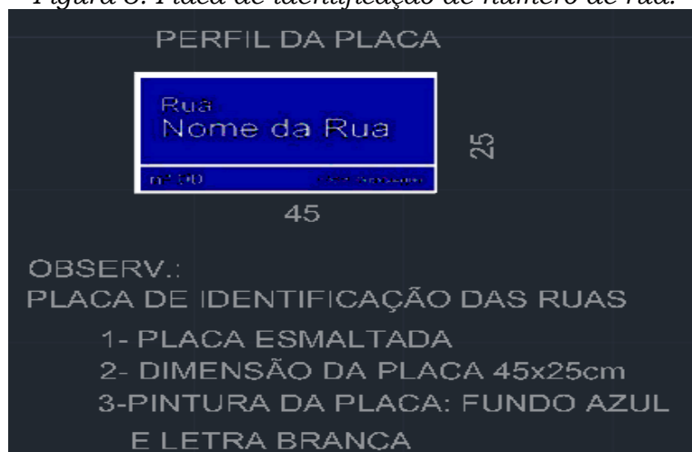
Figura 3. Placa de identificação de número de rua.
