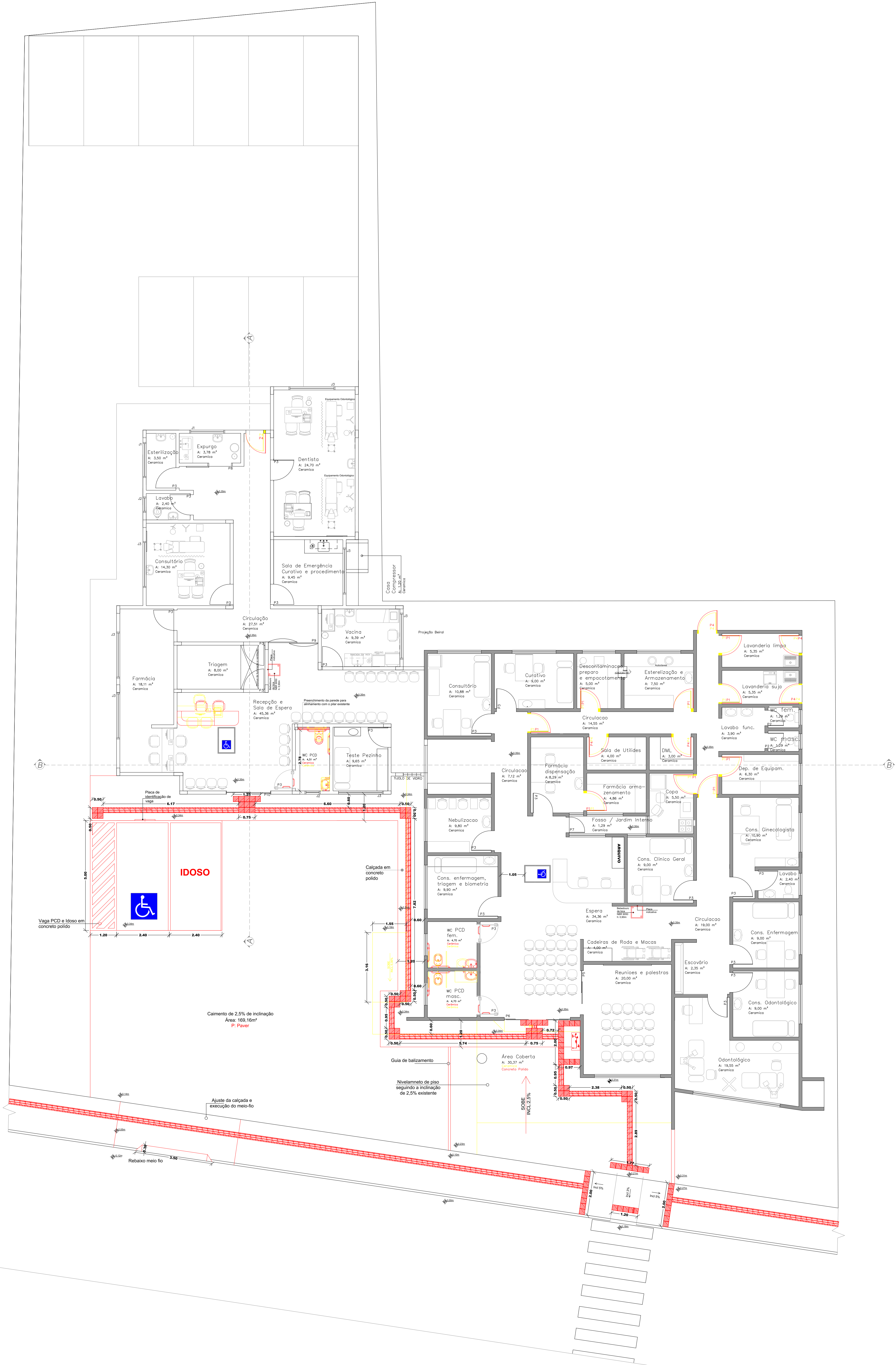
PLANTA BAIXA - Á DEMOLIR/ Á CONSTRUIR ESC: 1/75
