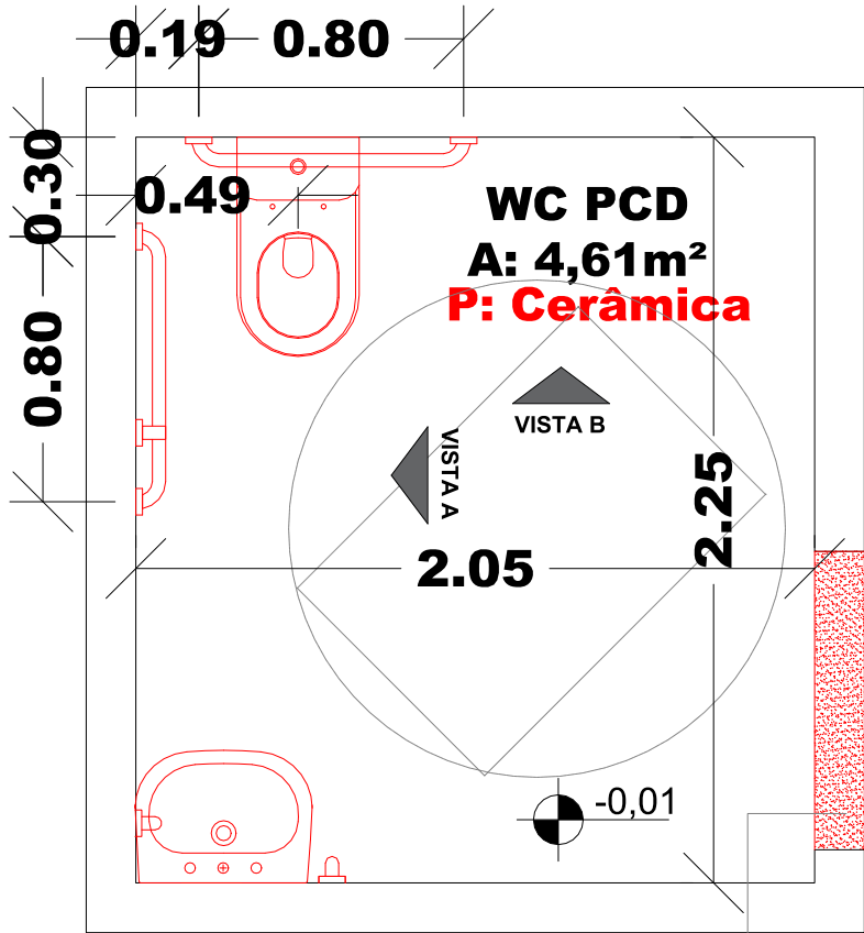
DETALHE 01 ESC:1/25
