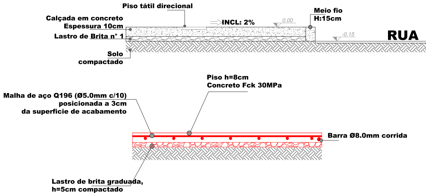
DETALHE 03 ESC:1/25
