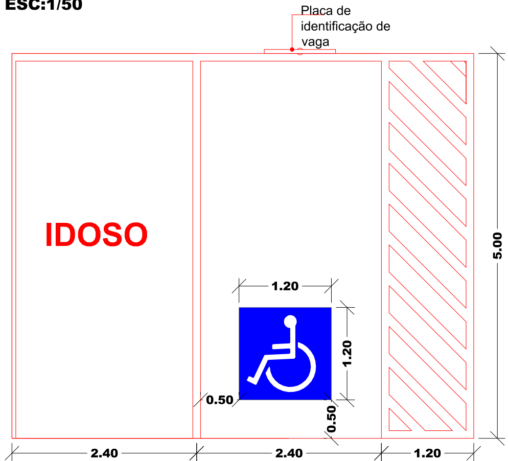
DETALHE 02 ESC:1/50
