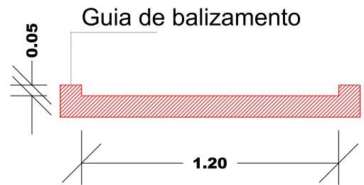
DETALHE 05 ESC:1/25
