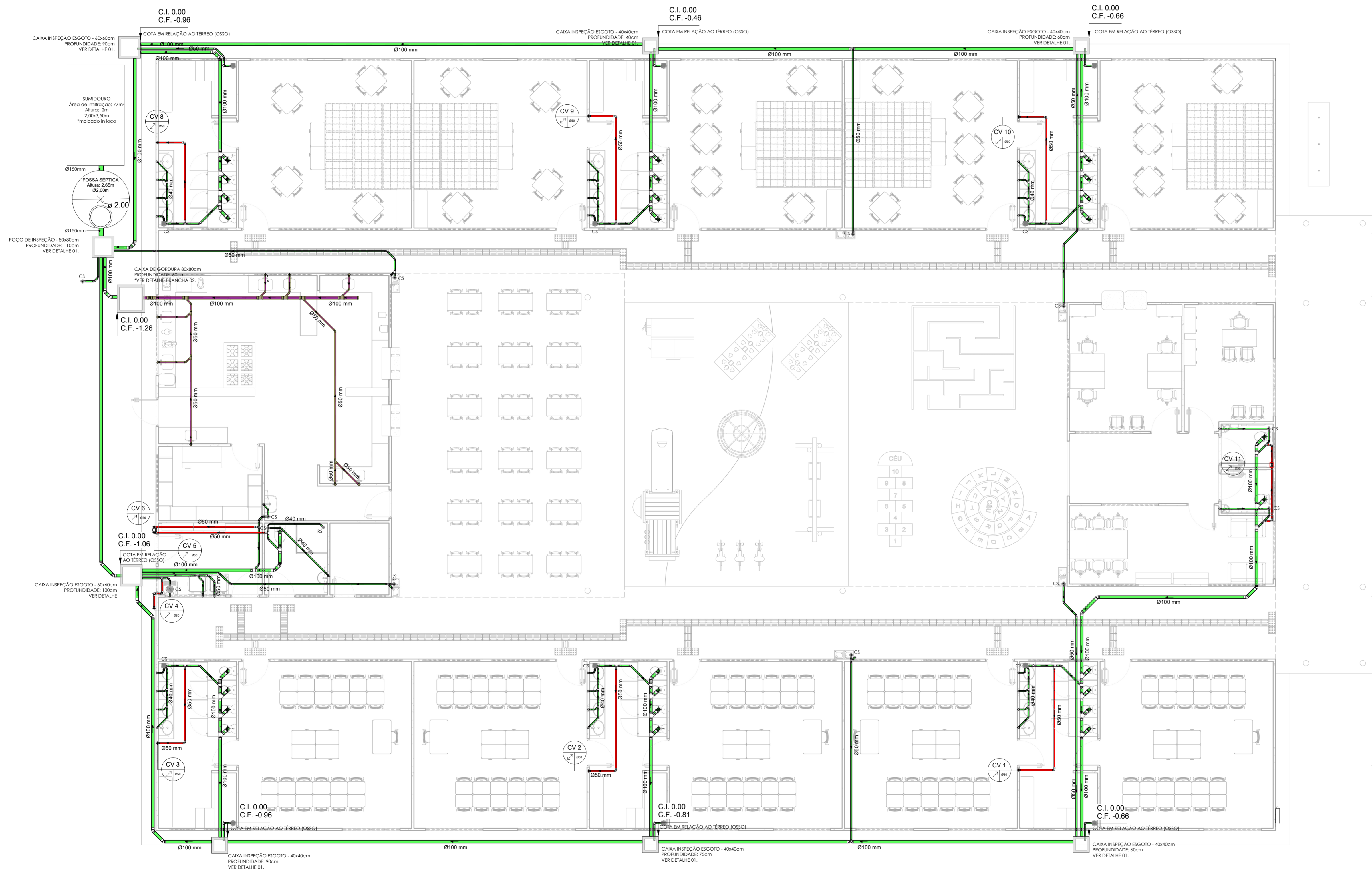
PLANTA BAIXA - TÉRREO ESCALA 1:75
