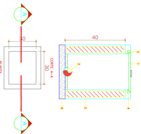
DET. CAIXA DE RECARGA DE ÁGUAS PLUVIAIS (SEM ESCALA)
