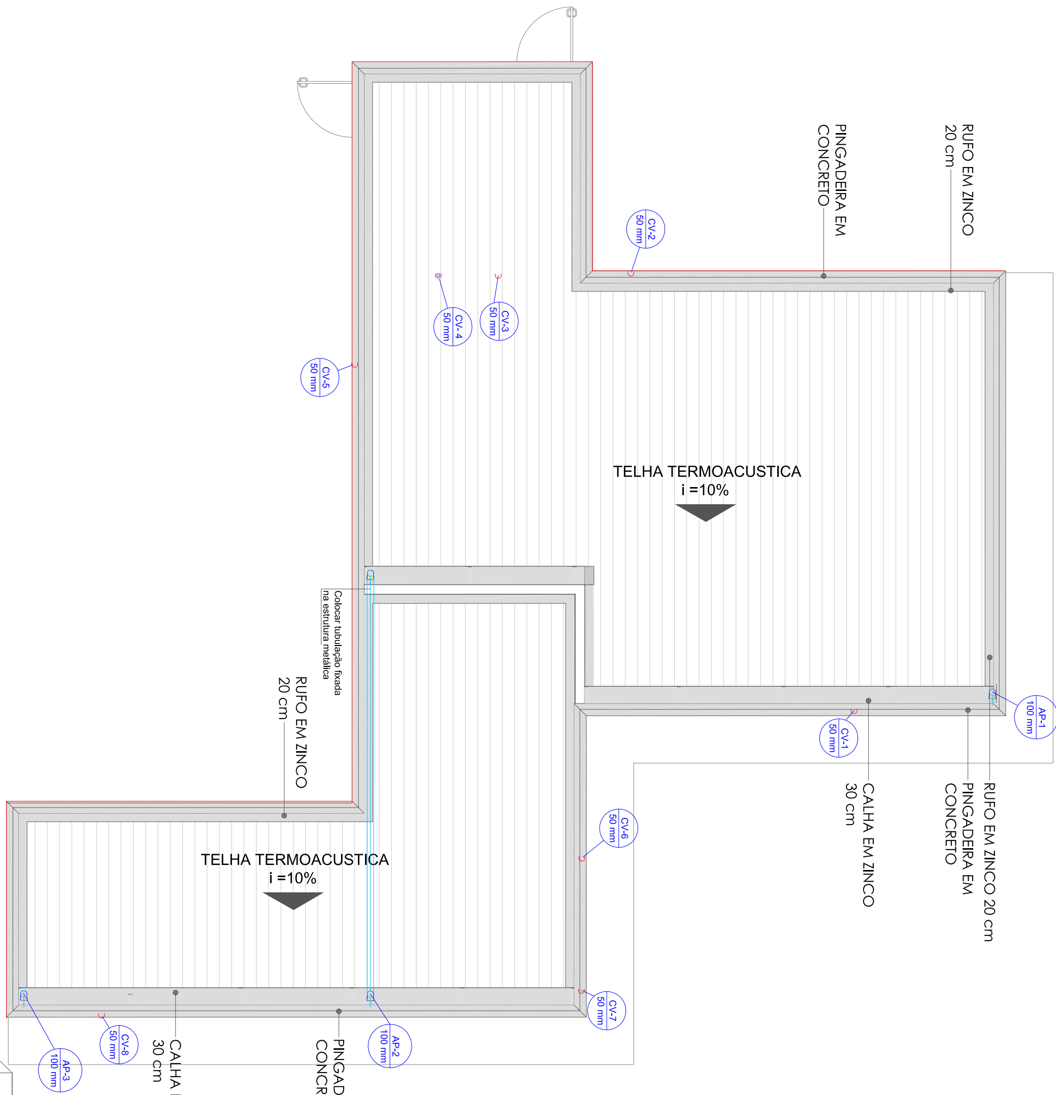
ESGOTO PLUVIAL E SANITÁRIO - NÍVEL SUPERIOR Escala 1:50
