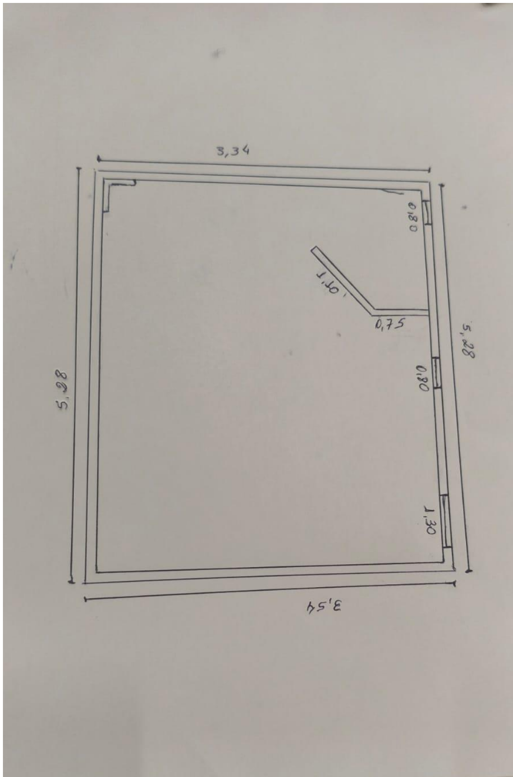
Figura 1 – Croqui do ambiente destinado à instalação do aparelho de Radiografia Digital (DR), com área aproximada de 17,64 m 2 .
