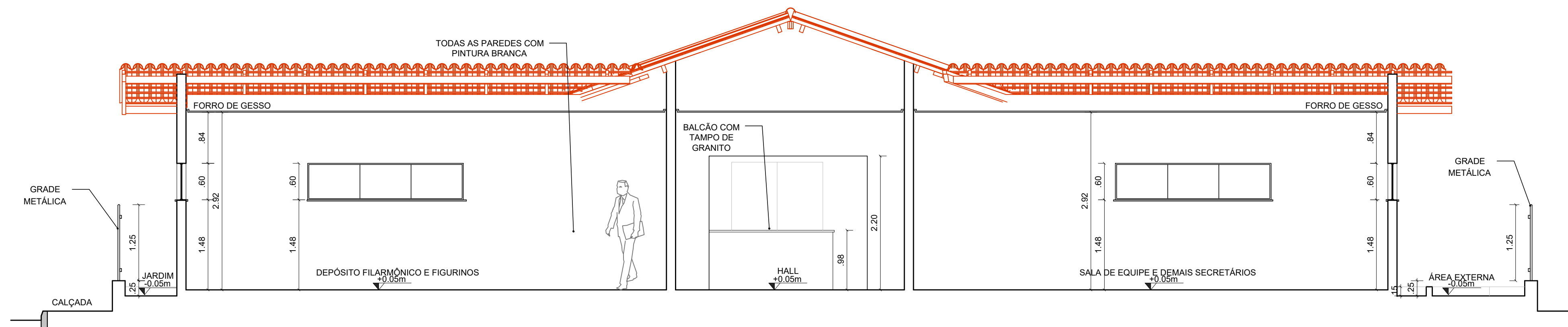
05 | CORTE AA' - CENTRO CULTURAL DO VAQUEIRO
