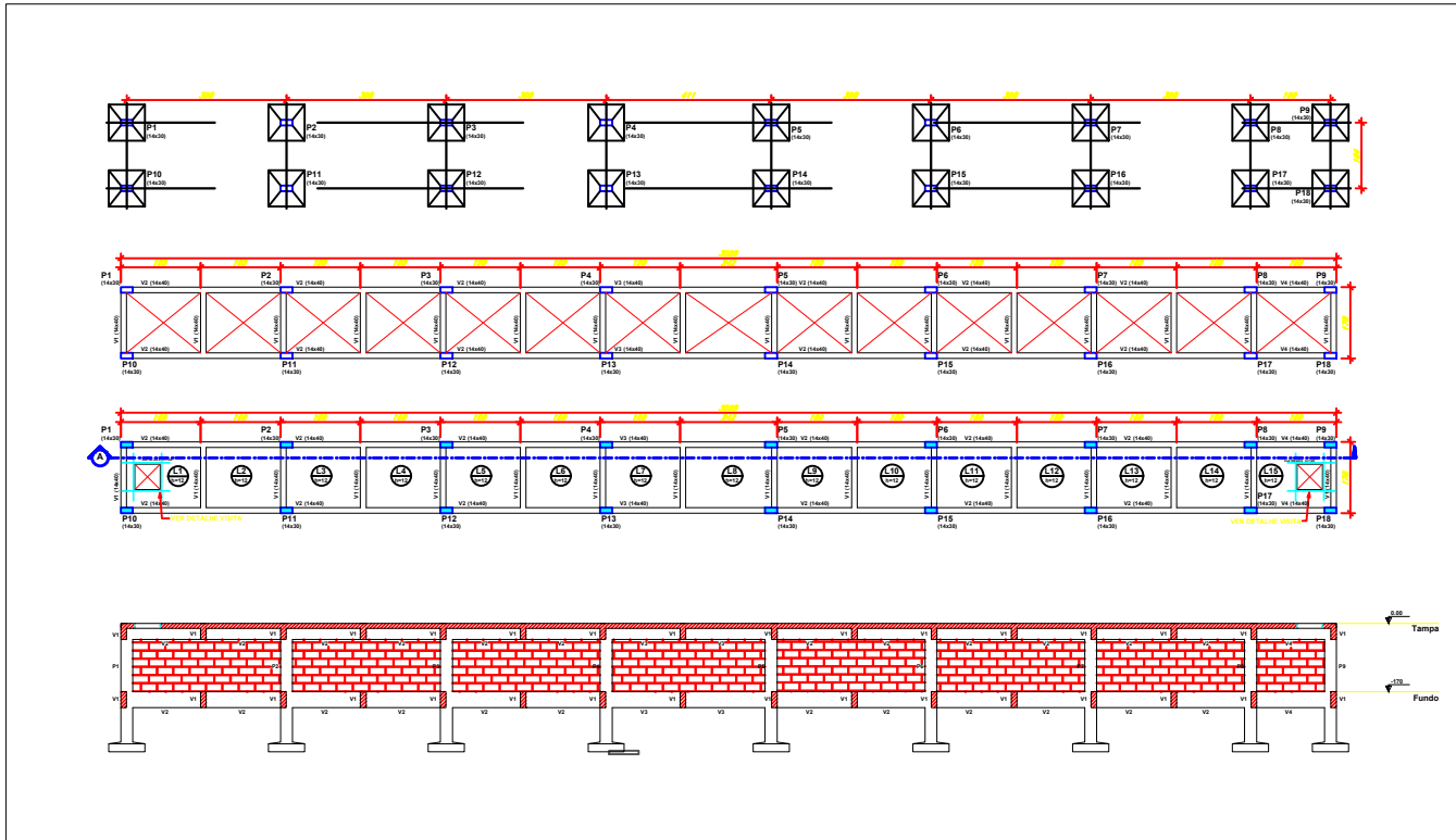
4 ESTRUTURAL - SUMIDOURO SEM ESCALA
