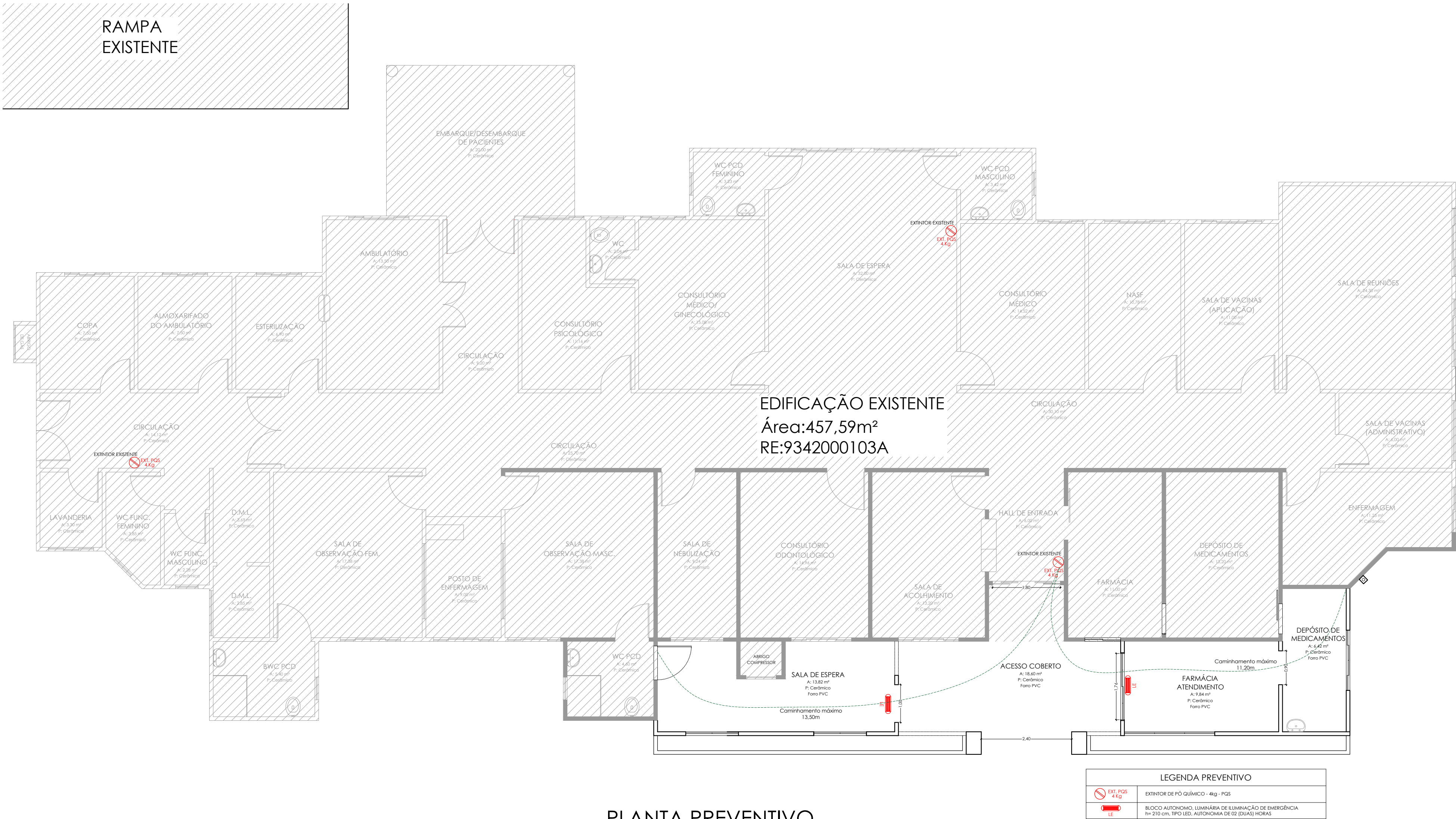
PLANTA PREVENTIVO ESCALA 1/75
