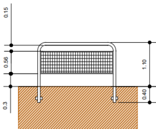
Corte - Gradil tipo 1
