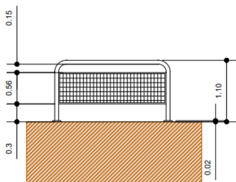
Corte - Gradil tipo 2
