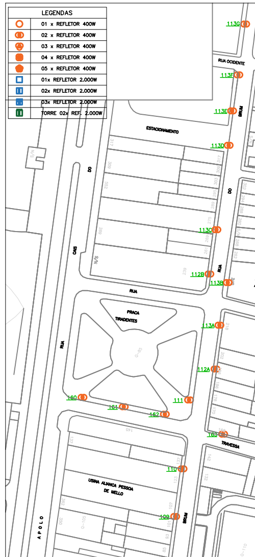
12 PLANTA DE LOCAÇÃO – RUA DO BRUM SEM ESCALA
