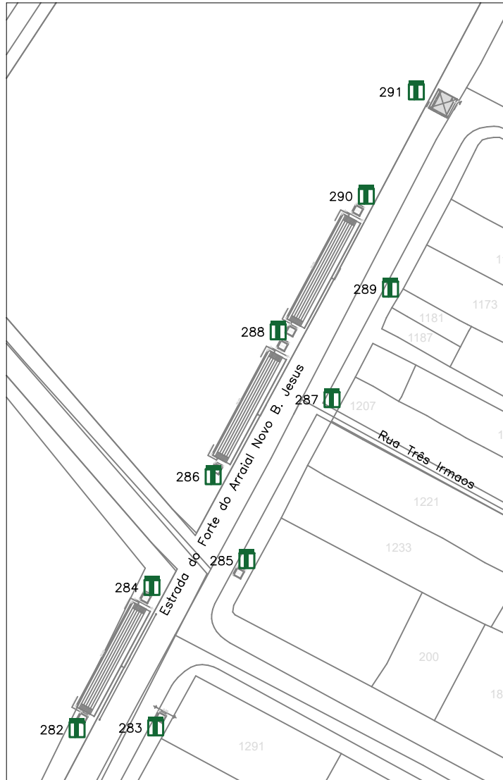
14 PLANTA DE LOCAÇÃO – ESTRADA DO FORTÉ (AVENIDA DO FORTÉ) SEM ESCALA
