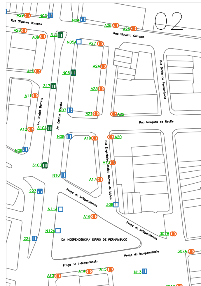
16 PLANTA DE LOCAÇÃO – TRECHO PRAÇA DA INDEPENDÊNCIA SEM ESCALA
