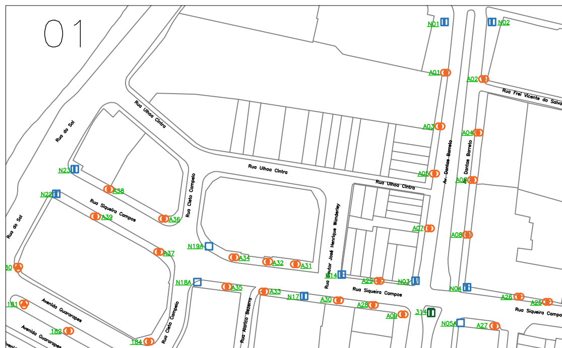
15 PLANTA DE LOCAÇÃO - TRECHO DA SIQUEIRA CAMPOS SEM ESCALA
