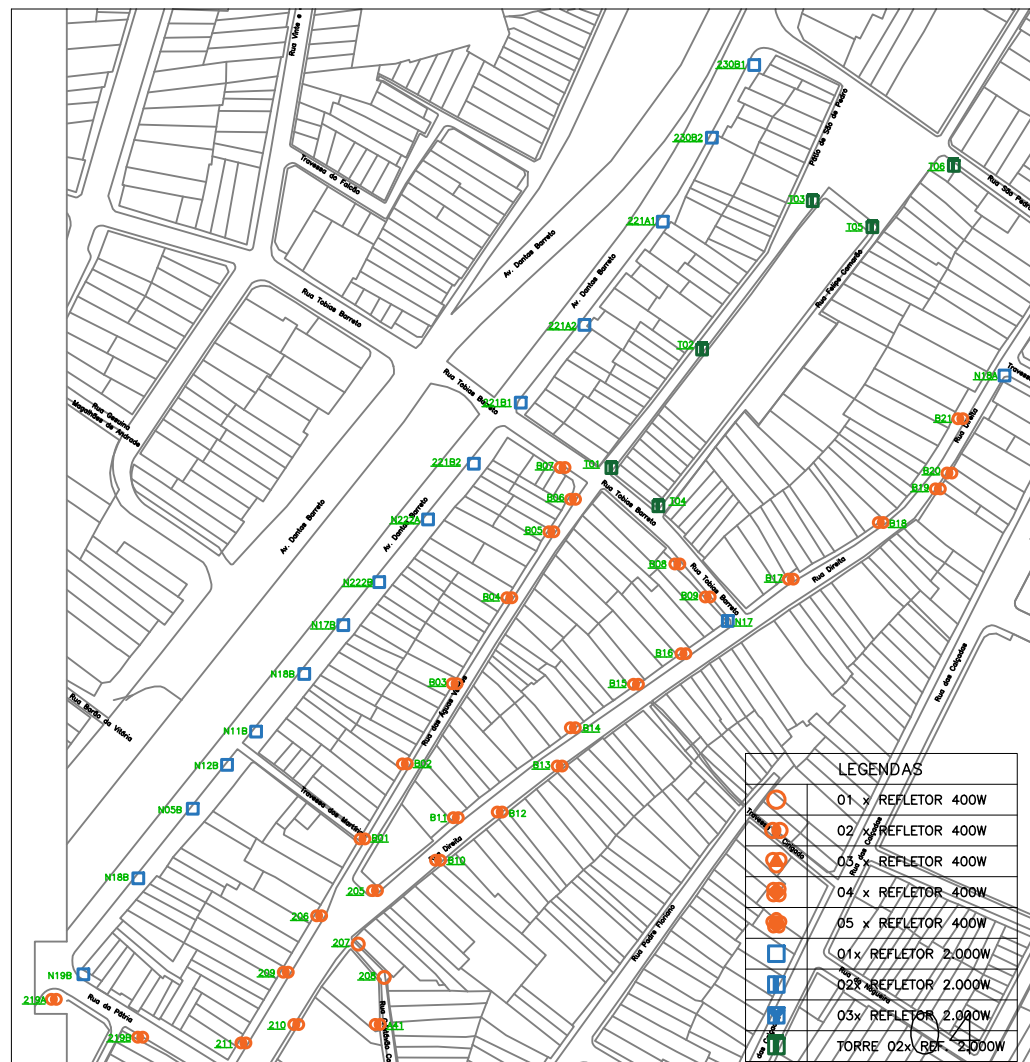
18 PLANTA DE LOCAÇÃO – TRECHO DO PÁTIO DE SÃO PEDRO SEM ESCALA
