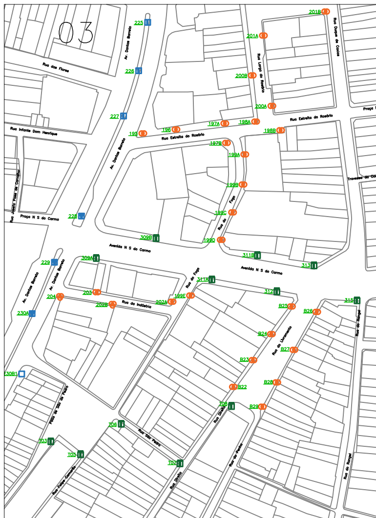
17 PLANTA DE LOCAÇÃO – TRECHO DA NOSSA SENHORA DO CARMO SEM ESCALA
