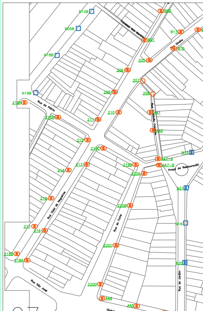
3 PLANTA DE LOCAÇÃO – RUA VIDAL DE NEGREIROS SEM ESCALA
