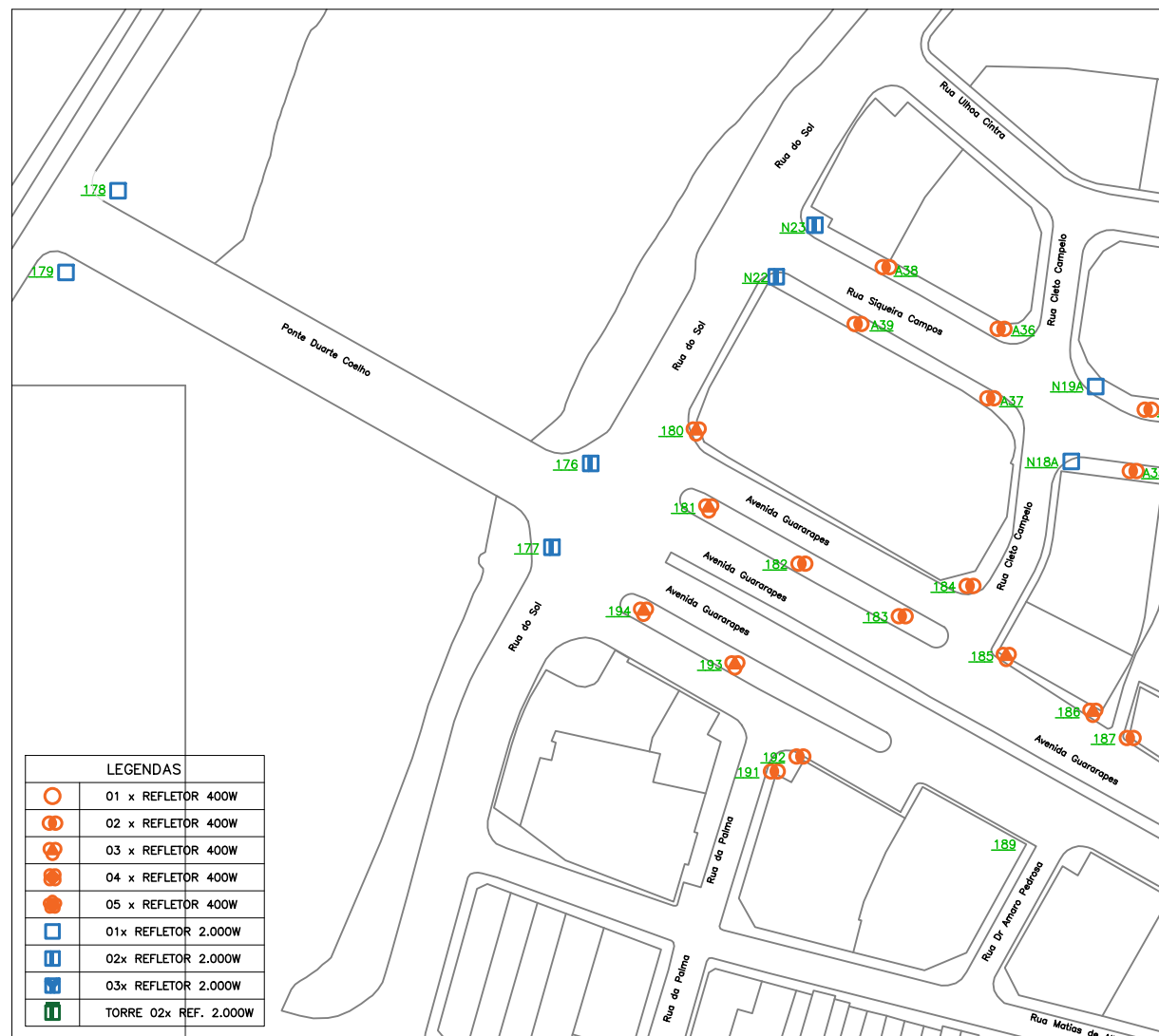
4 PLANTA DE LOCAÇÃO – AVENIDA GUARARAPES SEM ESCALA
