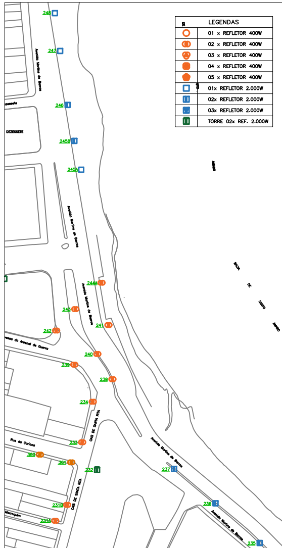
7 PLANTA DE LOCAÇÃO – MARTINS DE BARROS SEM ESCALA
