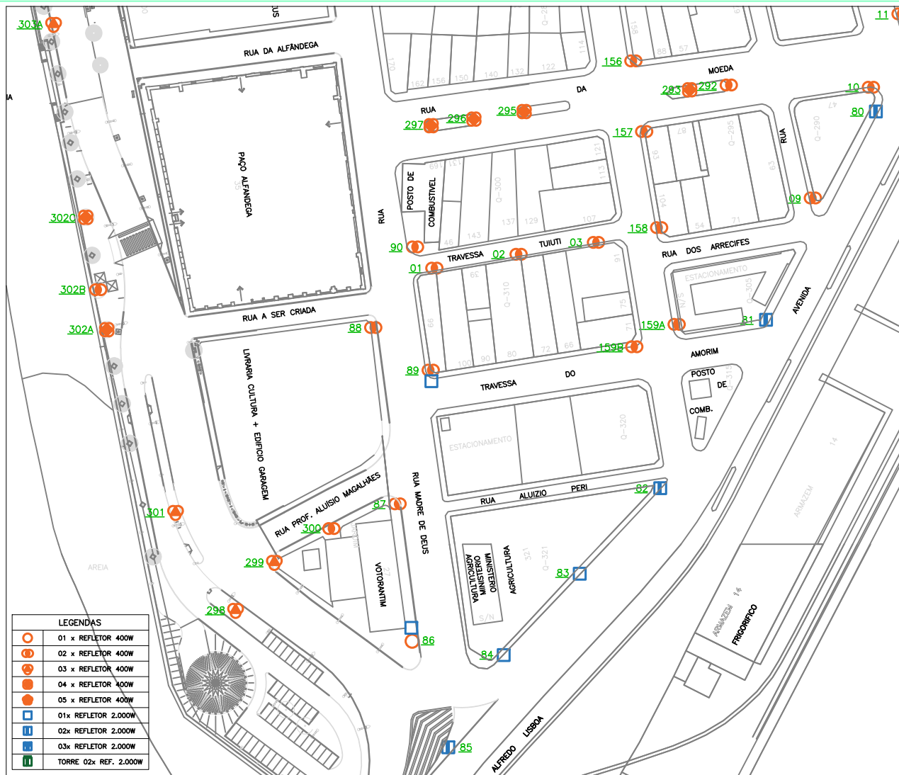
9 PLANTA DE LOCAÇÃO – RUA MADRE DE DEUS SEM ESCALA
