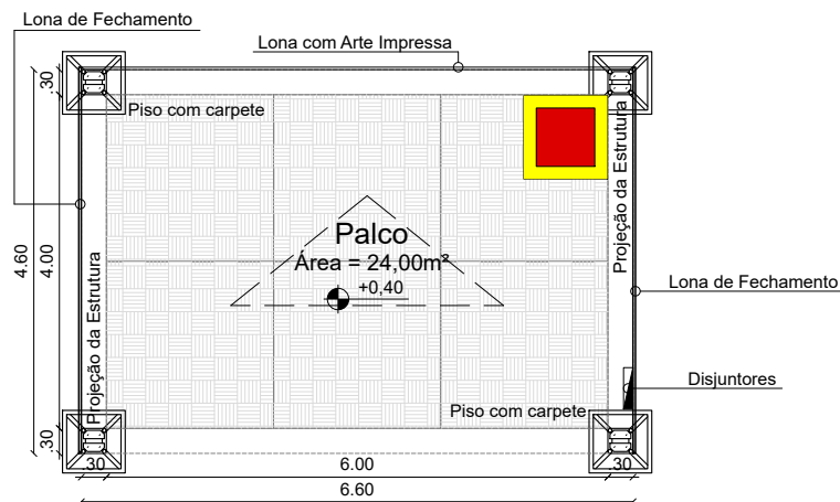
1 PLANTA BAIXA – PALCO CORREDOR 6,00x4,00m ESCALA – 1:100
