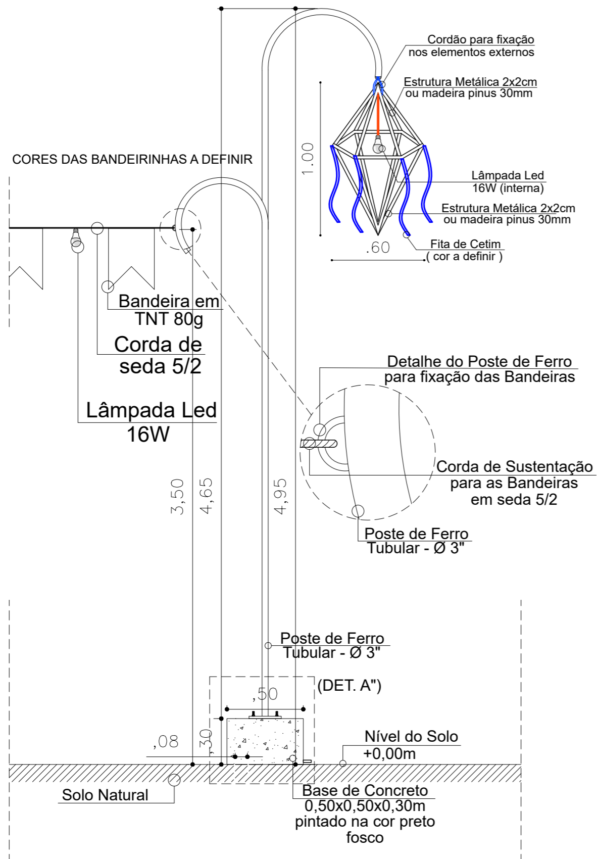
9 ELEVÇÃO FRONTAL – BASE BANDEIRINHAS – SÍTI0 TRINDADE ESCALA – 1:25
