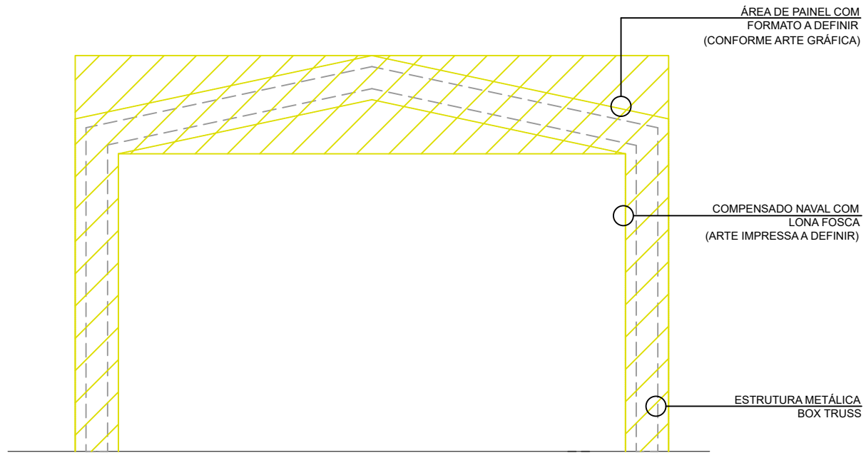
1 VISTA FRONTAL – PAVILHÃO PÉ DE SERRA – ELEMENTO INTERATIVO ESCALA – 1:50
