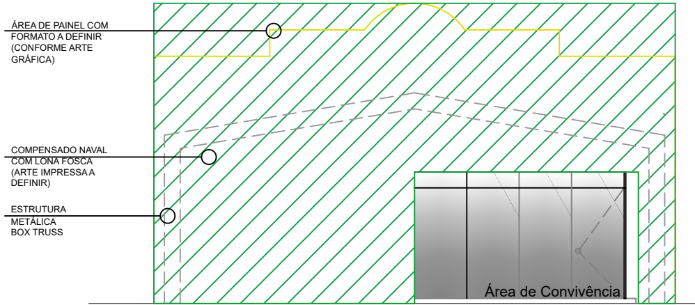
4 VISTA FRONTAL – MÓDULO ADMINISTRATIVO – ELEMENTO INTERATIVO ESCALA – 1:100
