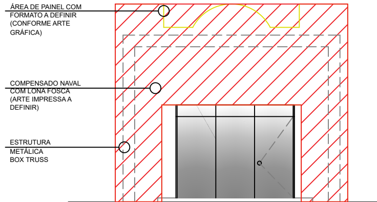
5 VISTA FRONTAL – MÓDULO SIMPLES – ELEMENTO INTERATIVO ESCALA – 1:100
