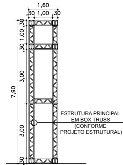
2 VISTA LATERAL – PÓRTICO (ESTRUTURA) ESCALA – 1:125
