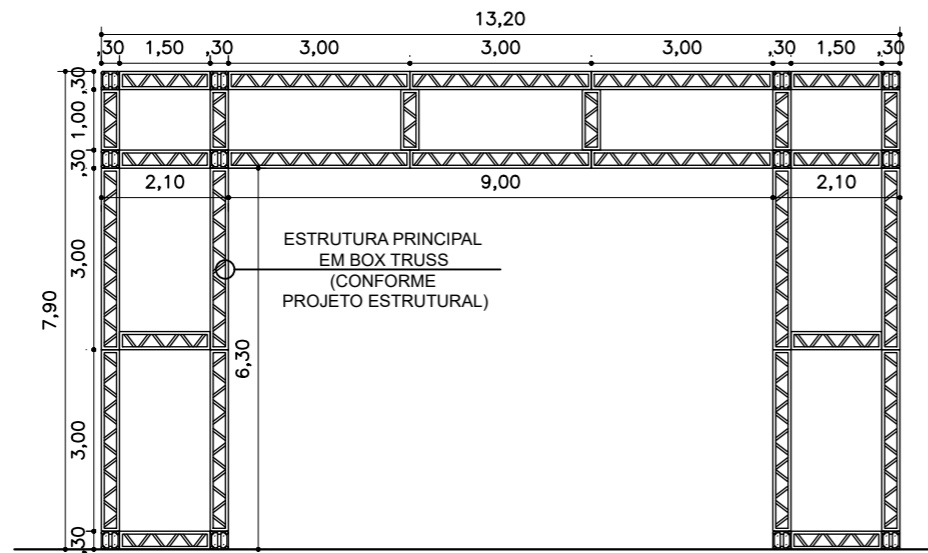
1 VISTA FRONTAL – PÓRTICO DE ENTRADA – (ESTRUTURA) ESCALA – 1:125
