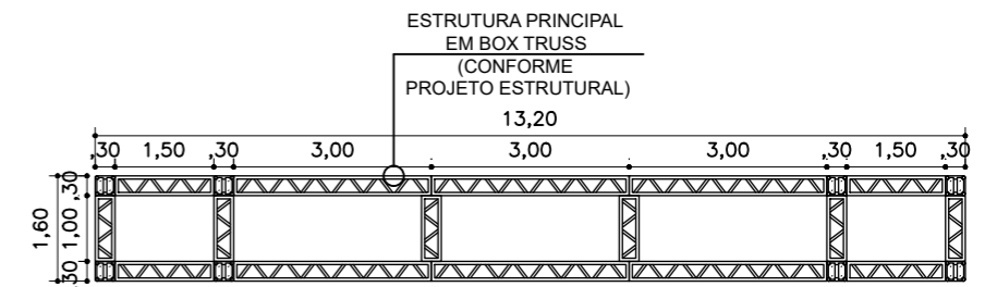
3 PLANTA BAIXA – PÓRTICO – BAIRRO DO RECIFE (ESTRUTURA) ESCALA – 1:125
