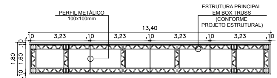
6 PLANTA BAIXA – PÓRTICO – BAIRRO DO RECIFE (PERFIL METÁLICO) ESCALA – 1:125
