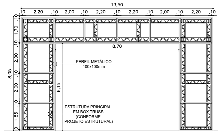
4 VISTA FRONTAL – PÓRTICO DE ENTRADA – (PERFIL METÁLICO) ESCALA – 1:125
