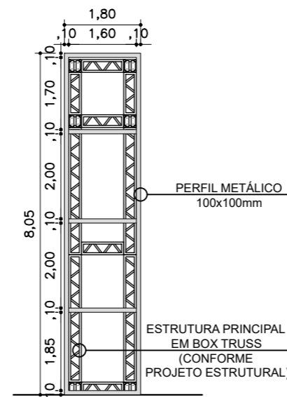
5 VISTA LATERAL – PÓRTICO – (PERFIL METÁLICO) ESCALA – 1:125
