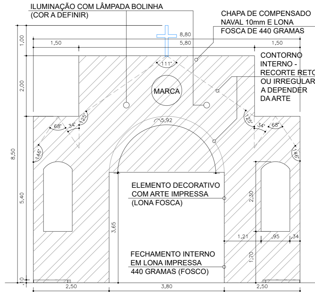
5 VISTA POSTERIOR – ELEMENTO PÓRTICO – PÁTIO SÃO PEDRO ESCALA – 1:75
