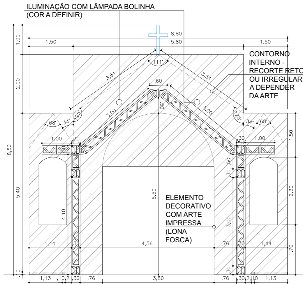
4 VISTA ESTRUTURA – ELEMENTO PÓRTICO – PÁTIO SÃO PEDRO ESCALA – 1:75
