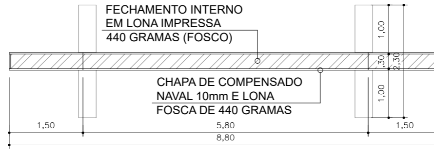
2 VISTA SUPERIOR – ELEMENTO PÓRTICO – PÁTIO SÃO PEDRO ESCALA – 1:75
