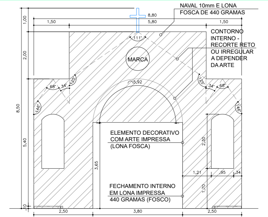
3 VISTA FRONTAL – ELEMENTO PÓRTICO – PÁTIO SÃO PEDRO ESCALA – 1:100
