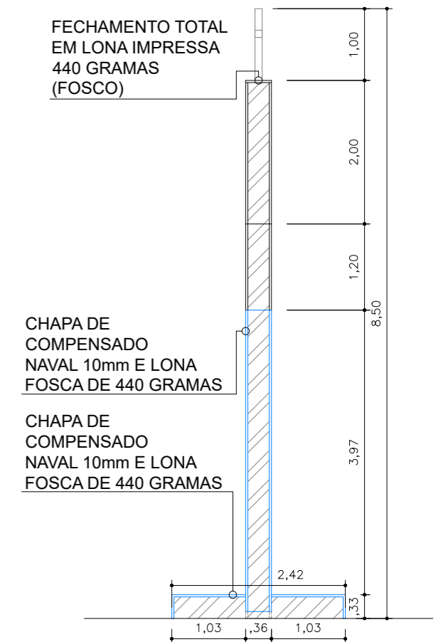
6 VISTA LATERAL – ELEMENTO PÓRTICO ESCALA – 1:75
