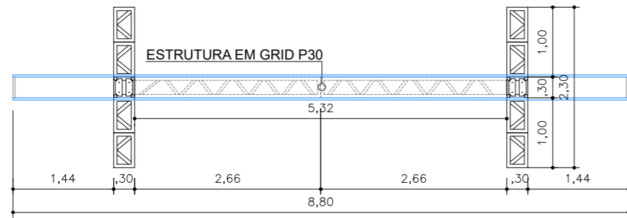
1 PLANTA BAIXA – ELEMENTO PÓRTICO – PÁTIO SÃO PEDRO (ESTRUTURA) ESCALA – 1:75
