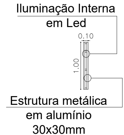
VISTA LATERAL – DISPLAY DA LOGOMARCA
