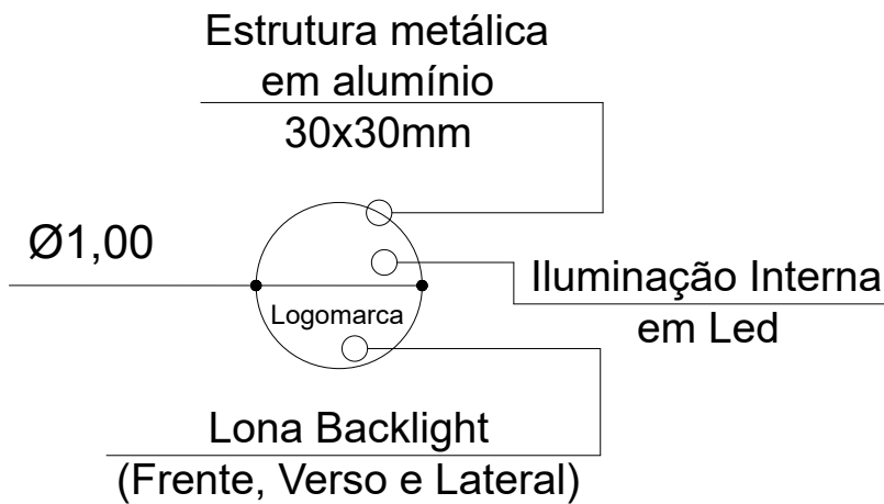
VISTA FRONTAL – DISPLAY DA LOGOMARCA – SALA DE REBOCO
