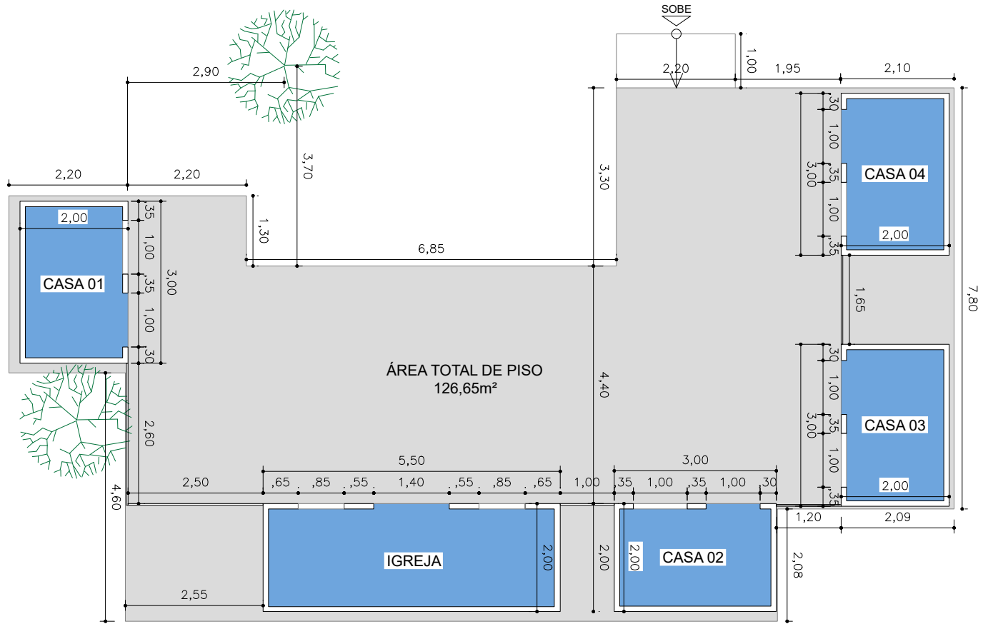
2 PLANTA BAIXA – VILA JUNINA – SÍTIO TRINDADE ESCALA – 1:100
