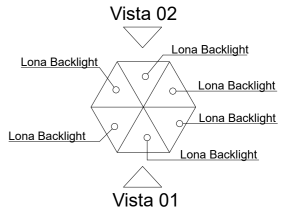
4 PLANTA BAIXA SUPERIOR – BALÕES AÉREOS LUMINOSOS ESCALA – 1:25
