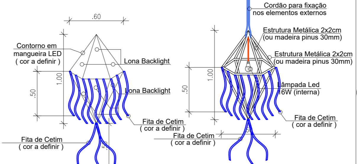
3 DETALHAMENTO – BALÕES AÉREOS LUMINOSOS ESCALA – 1:25
