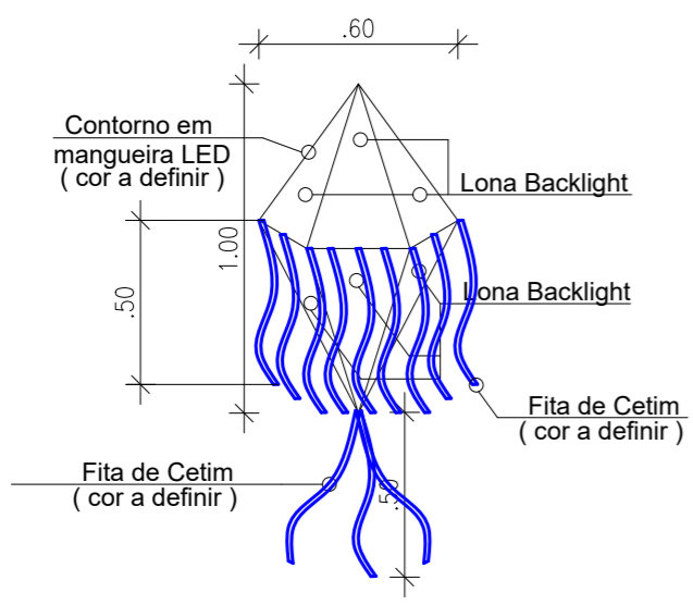
2 DETALHAMENTO – BALÕES AÉREOS LUMINOSOS ESCALA – 1:25
