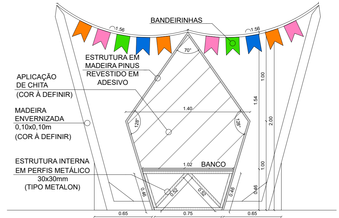
2 VISTA FRONTAL – BANCO BALÃO INTERATIVO – SÃO JOÃO (ESTRUTURA) ESCALA – 1:25
