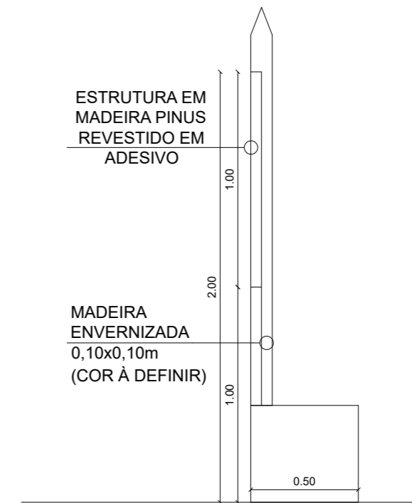
4 VISTA LATERAL – BANCO BALÃO INTERATIVO – SÃO JOÃO ESCALA – 1:25
