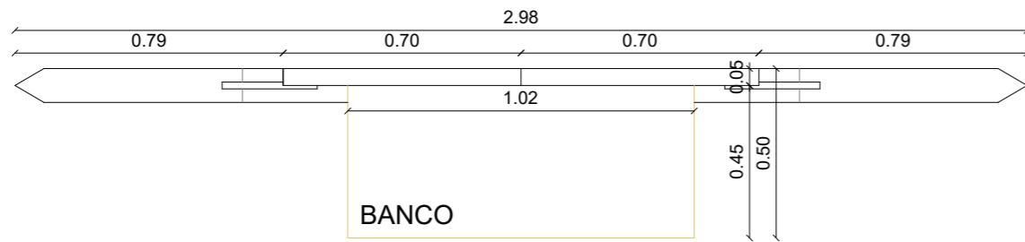
1 PLANTA BAIXA – BANCO BALÃO INTERATIVO – SÃO JOÃO ESCALA – 1:20
