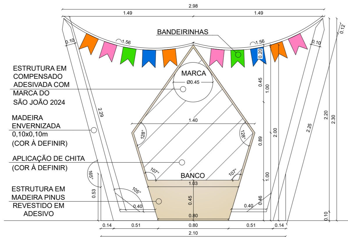
3 VISTA FRONTAL – BANCO BALÃO INTERATIVO – SÃO JOÃO ESCALA – 1:25
