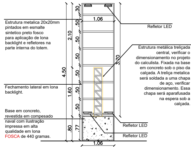
3 VISTA LATERAL DA ESTRUTURA – TOTEM DE SINALIZAÇÃO SEM ESCALA
