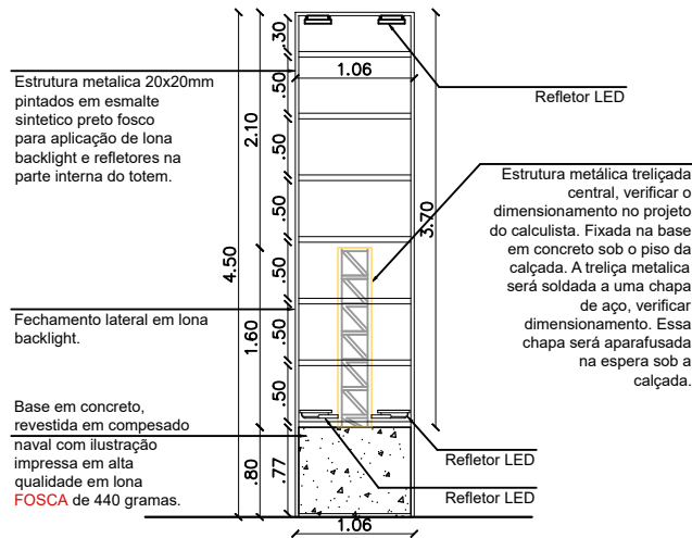
1 VISTA FRONTAL DA ESTRUTURA – TOTEM DE SINALIZAÇÃO SEM ESCALA
