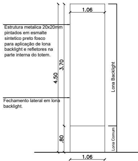
2 VISTA FRONTAL – TOTEM DE SINALIZAÇÃO SEM ESCALA
