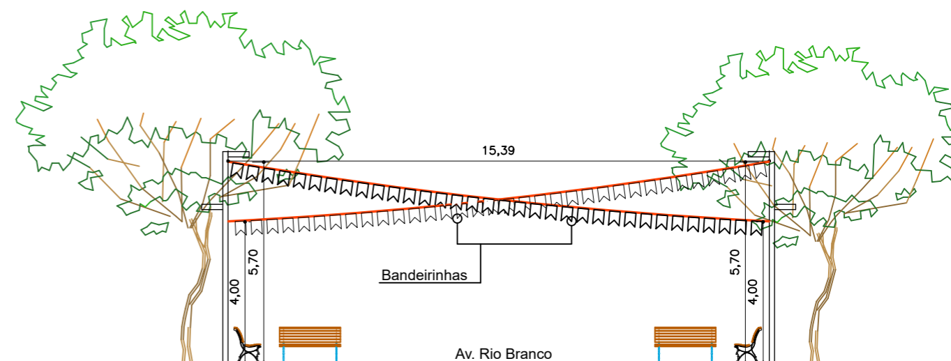
3 ELEVACÃO FRONTAL – DECORAÇÃO BANDEIRINHAS – AV. RIO BRANCO – SÃO JOÃO ESCALA – 1:150
