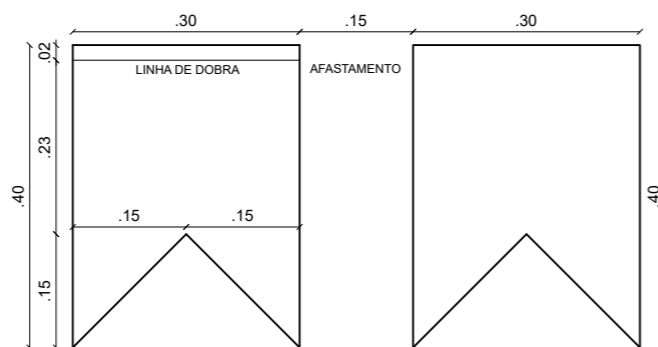
2 DETALHE – BANDEIRINHAS – AV. RIO BRANCO – SÃO JOÃO ESCALA – 1:10
