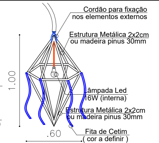
ESTRUTURAL – ELEMENTO BALÃO AÉREO
