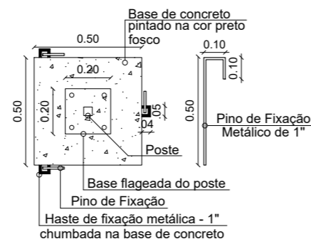
PLANTA BAIXA – ELEMENTO BASE BANDEIRINHAS
