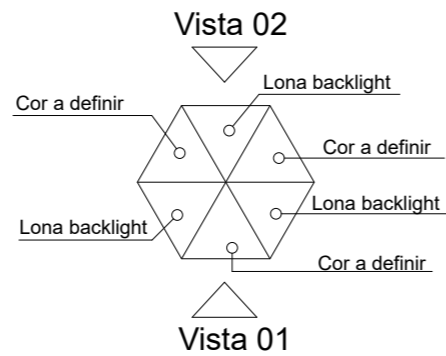
VISTA INFERIOR – ELEMENTO BALÃO AÉREO
