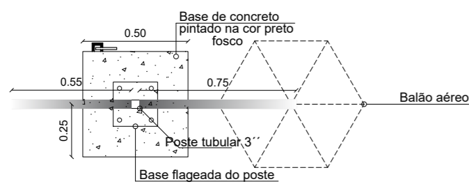
VISTA SUPERIOR – ELEMENTO BASE BANDEIRINHAS
