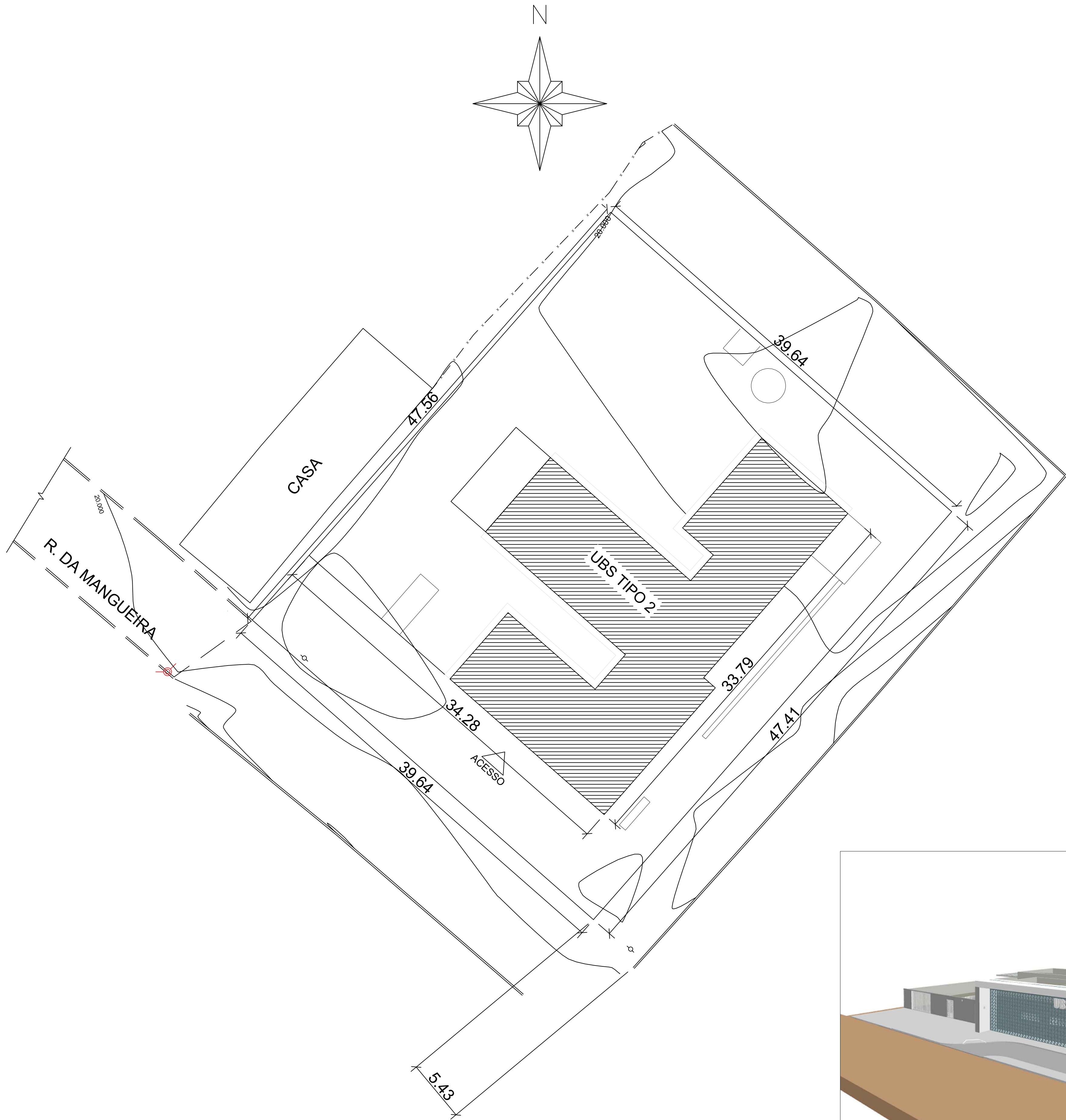
● PLANTA DE IMPLANTAÇÃO ESC 1:200
