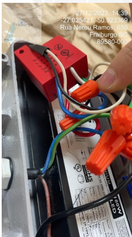
Figura 24 - Fiação interna do item 5
