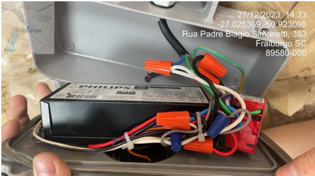
Figura 11 - Fiação interna do item 3
