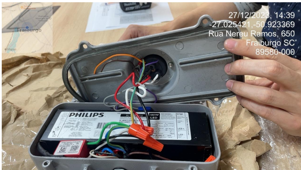
Figura 21 - Driver e fiação interna do item 5
