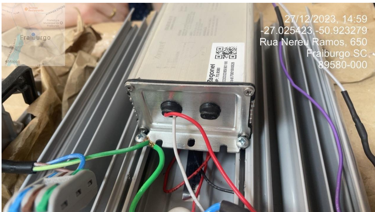
Figura 21 - Fiação do driver
