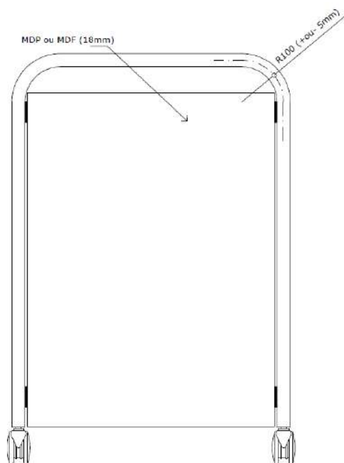
VISTA FRONTAL SEM ESCALA
