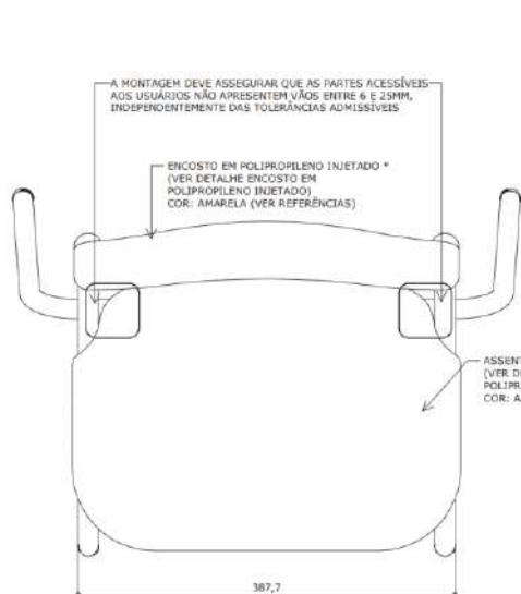
VISTA SUPERIOR ESC. 1 - 5
