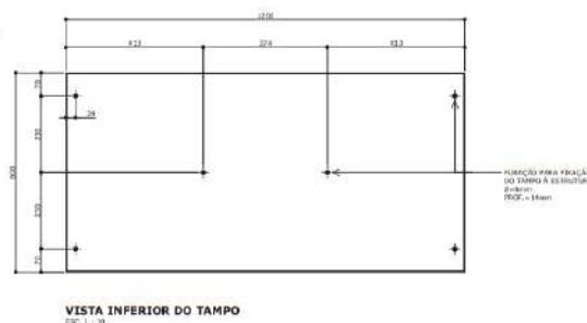
VISTA INFERIOR DO TAMPO ESC. 1 : 10
