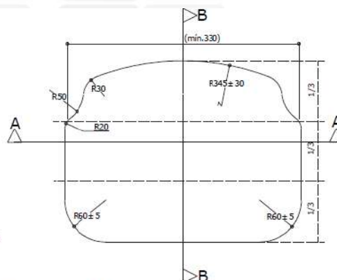
VISTA SUPERIOR ESC. 1 : 5
