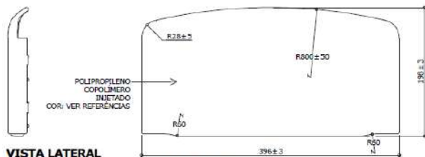
VISTA FRONTAL ESC. 1 : 5
