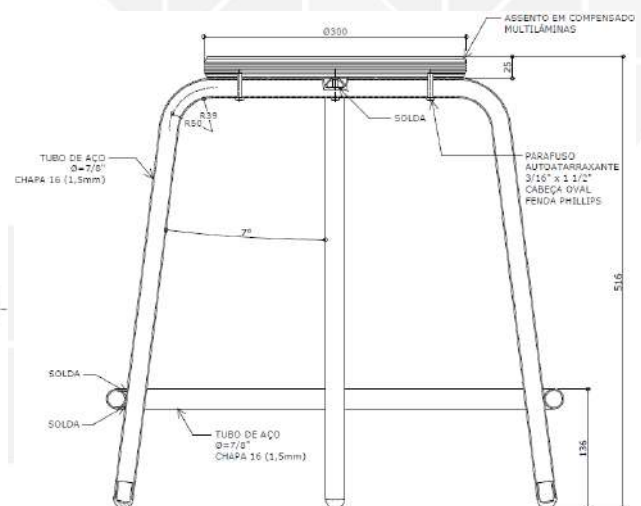
VISTA FRONTAL ESC. 1 : 5
