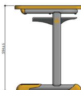
VISTA LATERAL ESC. 1 : 10
