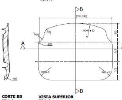
CORTE BB ESC. 1 : 5
