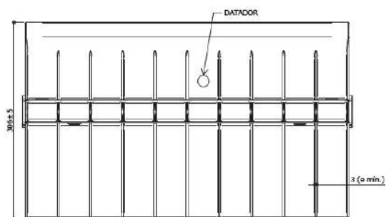
VISTA INFERIOR ESC. 1 : 5
