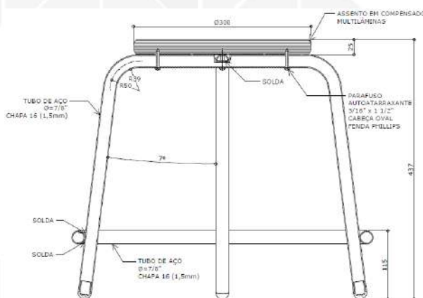
CORTE AA ESC. 1 : 5
