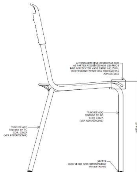
VISTA LATERAL PSC 1-5
