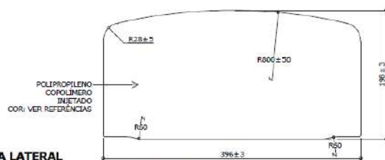
VISTA FRONTAL ESC. 1:1
