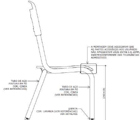
VISTA LATERAL ESC. 1 : 5
