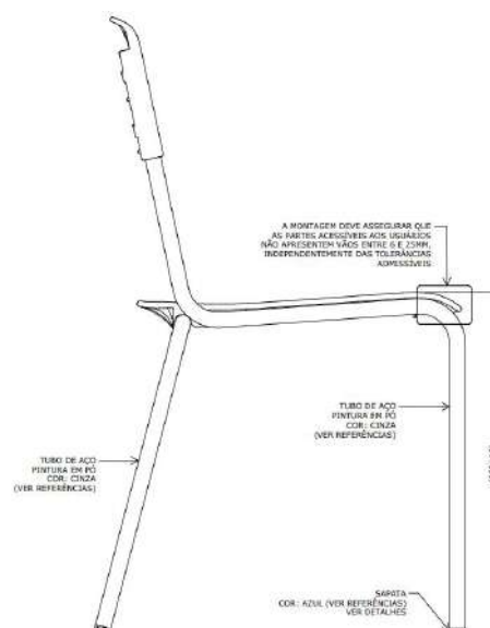
VISTA LATERAL FIG. 1-5
