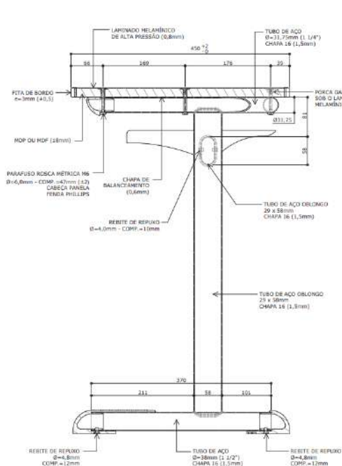
CORTE AA ESC. 1 : 5
