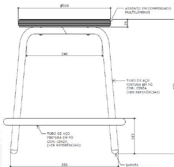
VISTA FRONTAL ESC. 1 : 5
