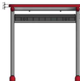
VISTA FRONTAL ESC. 1 : 10
