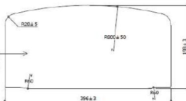
VISTA FRONTAL ESC. 1 : 5
