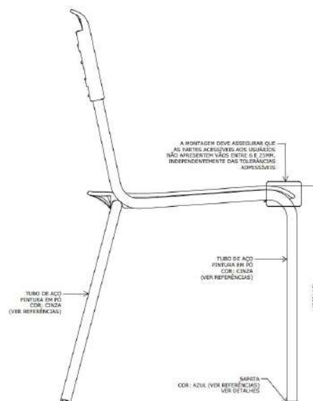
VISTA LATERAL ESC. 1 : 5
