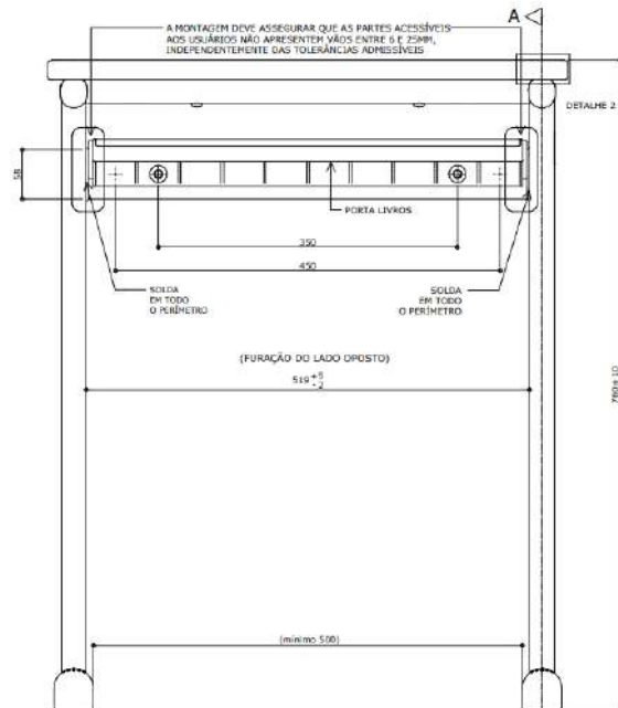
VISTA FRONTAL ESC. 1 : 5
