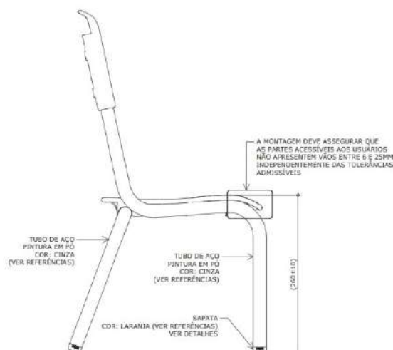
VISTA LATERAL ESC. 1 : 5
