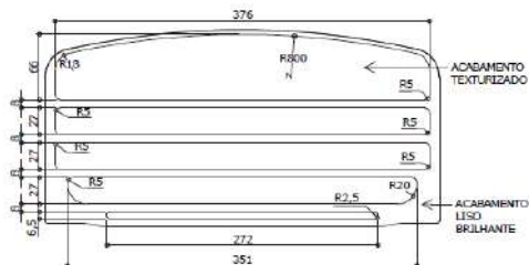
VISTA FRONTAL - ACABAMENTO ESC. 1 : 5
