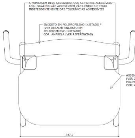
VISTA SUPERIOR ESC. 1 : 5
