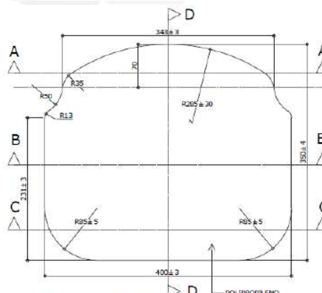
VISTA SUPERIOR ESC. 1 : 5
