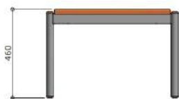
VISTA LATERAL ESC. 1 : 20
