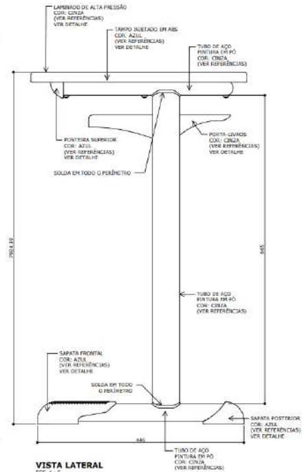
VISTA LATERAL ESC. 1 : 5
