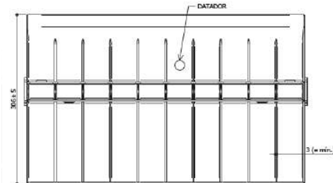
VISTA INFERIOR ESC. 1 : 5
