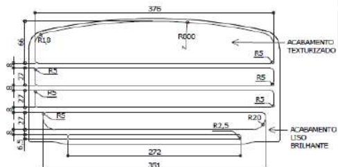
VISTA FRONTAL - ACABAMENTO ESC. 1 : 5
