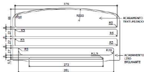
VISTA FRONTAL - ACABAMENTO PSC. 1 x 5
