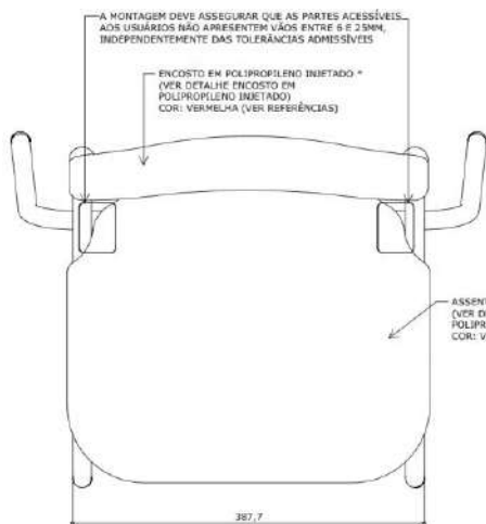
VISTA SUPERIOR ESC. 1 : 5
