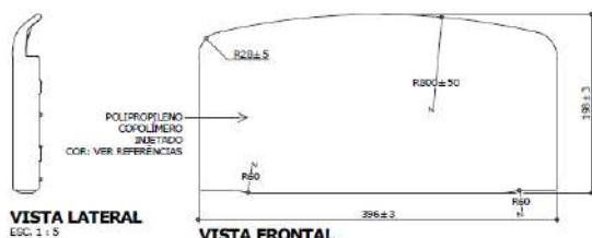
VISTA FRONTAL ESC. 1 : 5
