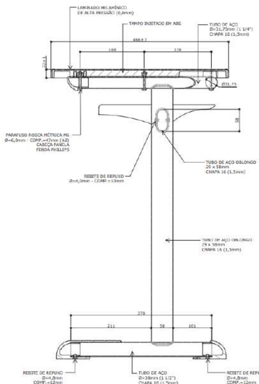
CORTE AA ESC. 1 : 5
