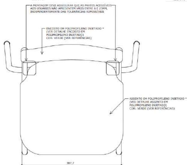
CORTE AA ESC. 1 : 5
