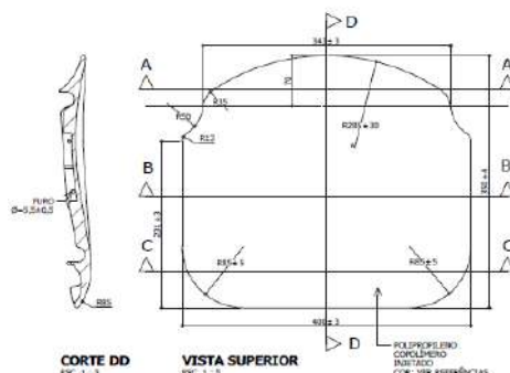
CORTE DD
