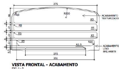
VISTA FRONTAL - ACABAMENTO ESC. 1 : 5
