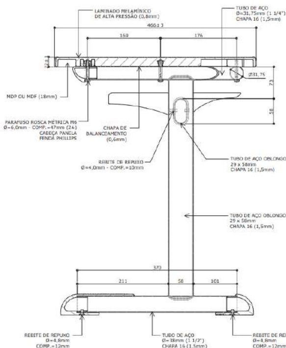
CORTE AA ESC. 1 : 5
