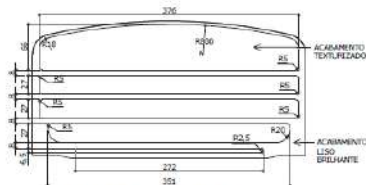
VISTA FRONTAL - ACABAMENTO ESC. 1 - 5
