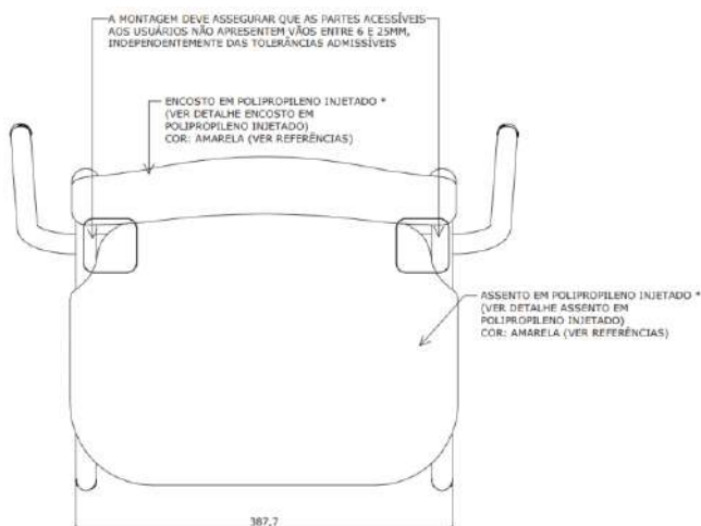
VISTA SUPERIOR ESC. 1 : 5
