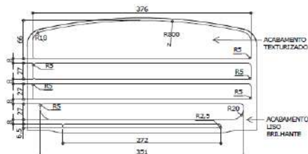
VISTA FRONTAL - ACABAMENTO ESC. 1 : 5
