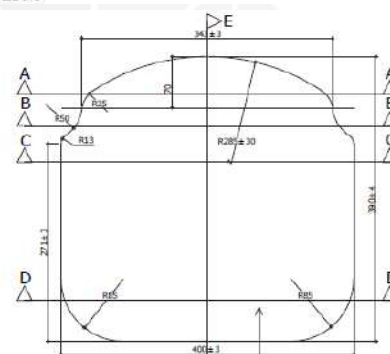
VISTA SUPERIOR ESC 1 : 5
