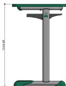
VISTA LATERAL ESC. 1 : 10
