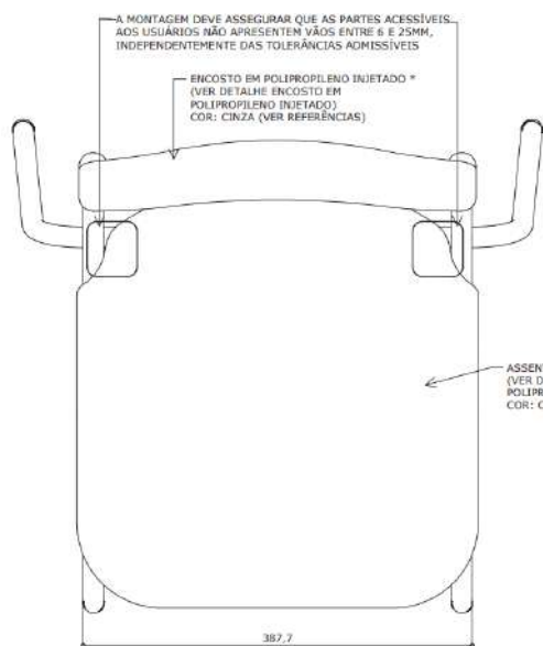
VISTA SUPERIOR ESC. 1 : 5
