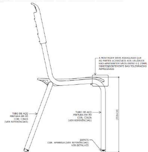
VISTA LATERAL ESC. 1 : 5
