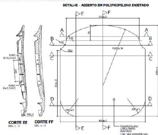
VISTA SUPERIOR ESC. 1 : 5
