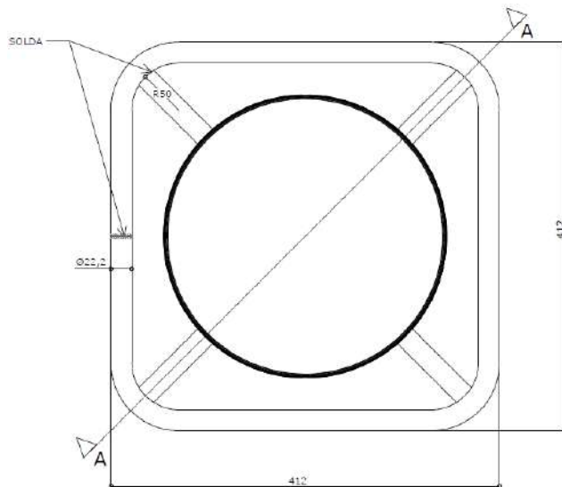
VISTA SUPERIOR ESC. 1 : 5
