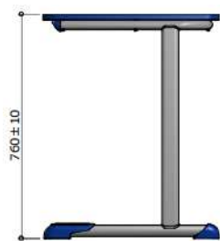
VISTA LATERAL ESC. 1 : 20
