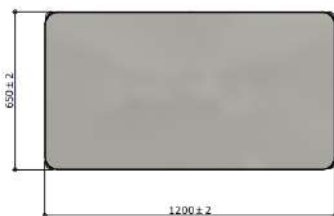
VISTA SUPERIOR ESC. 1 : 20
