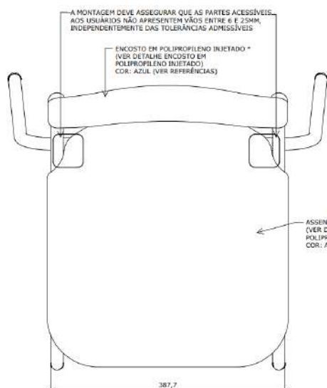
VISTA SUPERIOR ESC. 1 : 5
