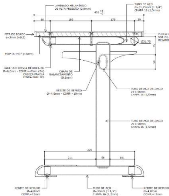
CORTE AA ESC. 1 : 5
