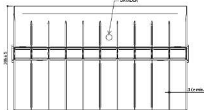
VISTA INFERIOR ESC. 1 : 5
