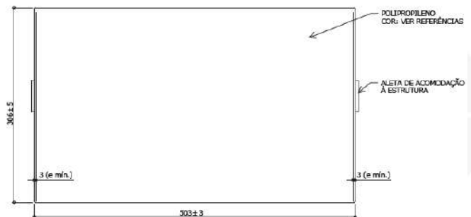
VISTA SUPERIOR ESC. 1 : 5
