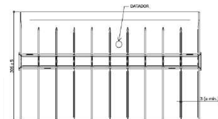
VISTA INFERIOR ESC. 1 : 5
