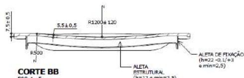
CORTE BB ESC. 115
