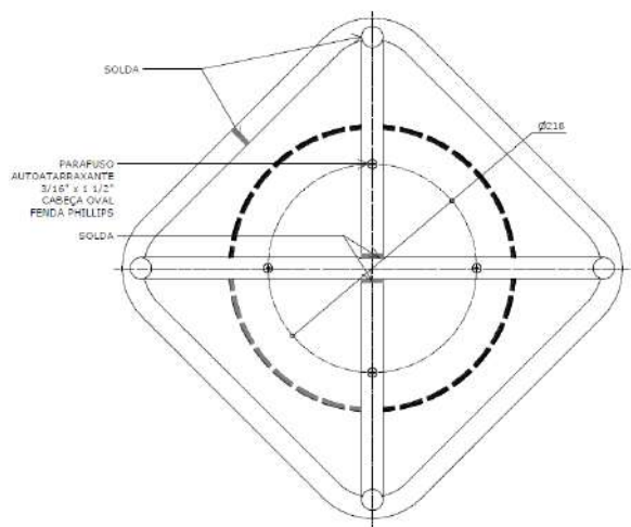
VISTA INFERIOR ESC. 1 : 5
