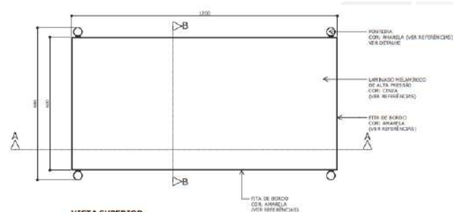
VISTA SUPERIOR ESC. 1 : 10
