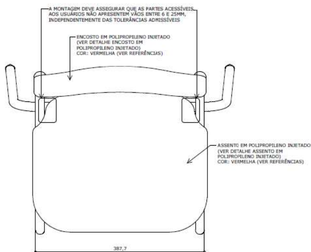
VISTA SUPERIOR ESC. 1 : 5
