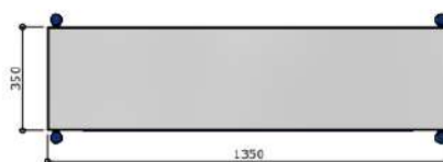
VISTA SUPERIOR ESC. 1 : 20
