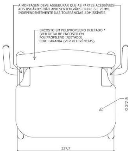
VISTA SUPERIOR ESC. 1 : 5
