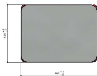
VISTA SUPERIOR ESC. 1 : 10
