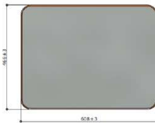
VISTA SUPERIOR ESC. 1 : 10
