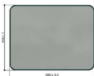
VISTA SUPERIOR ESC. 1 : 10
