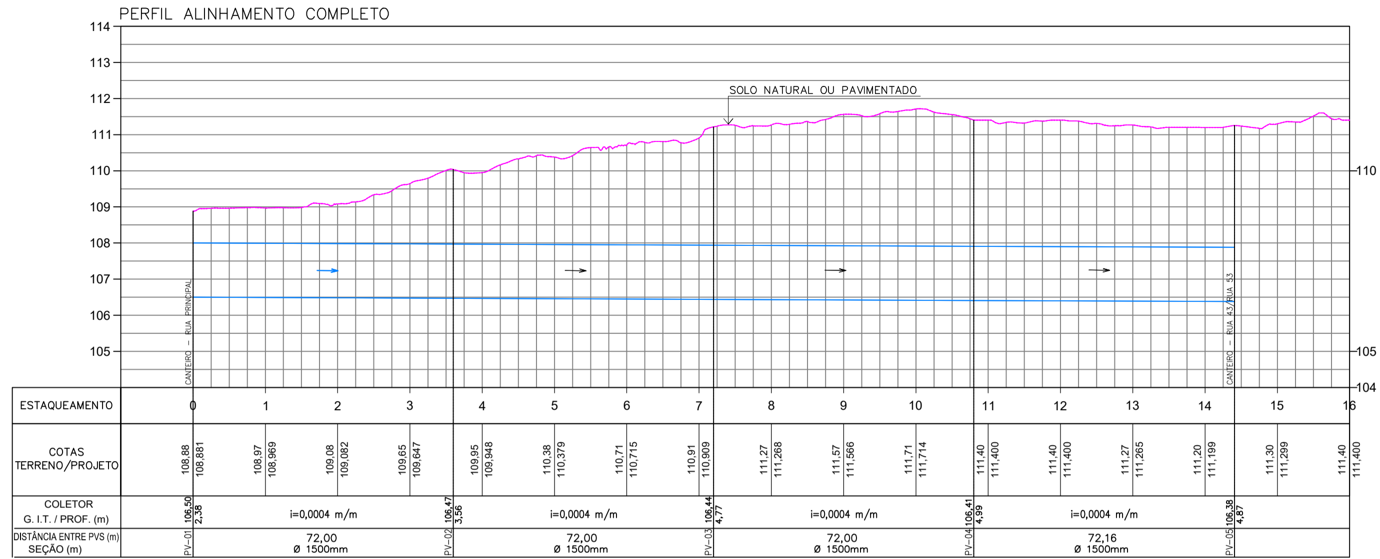
CANTEIRO CENTRAL - RUA PRINCIPAL ESCALAS: HORIZONTAL 1/1000; VERTICAL 1/100
