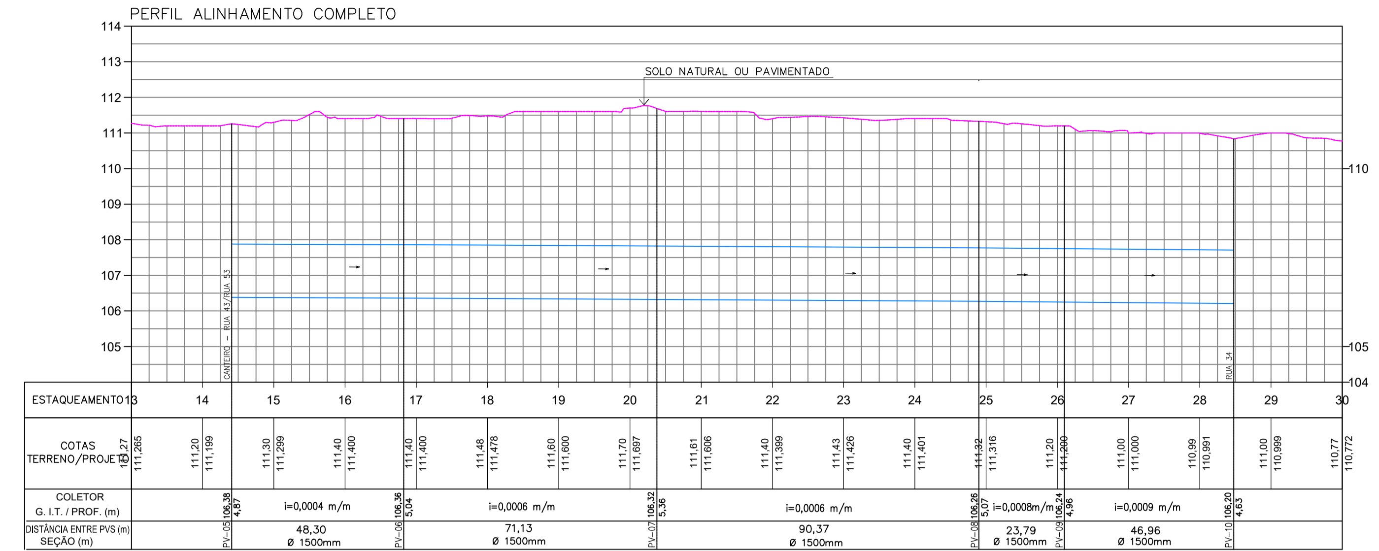
CANTEIRO CENTRAL - RUA 43 / RUA 53 ESCALAS: HORIZONTAL 1/1000; VERTICAL 1/100
