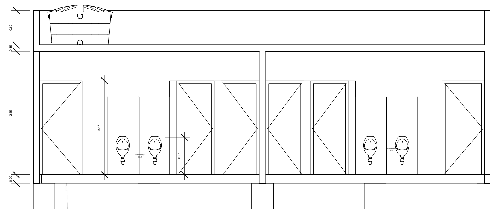
2 Corte AA'' 1 : 50
