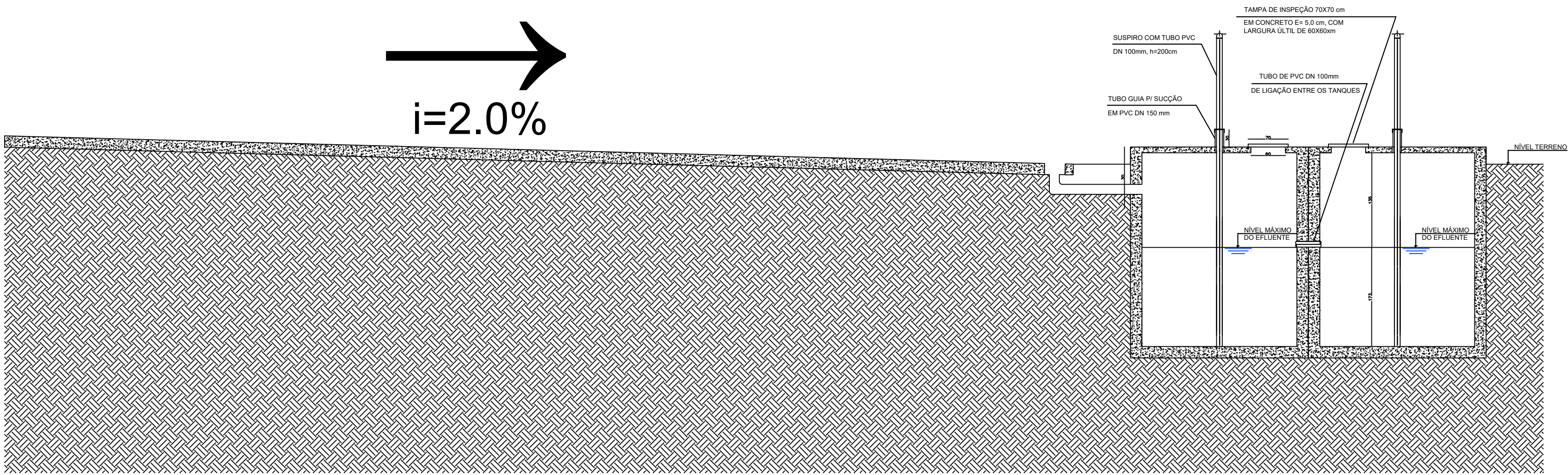
Corte B-B 1:100
