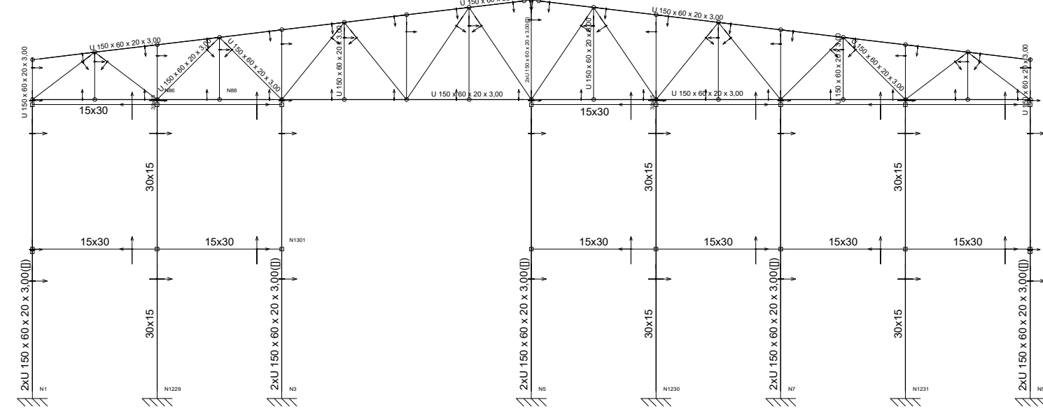
Oitão Fundo
