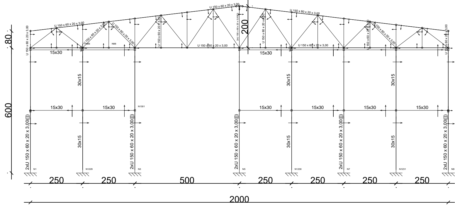
Oitão Frontal
