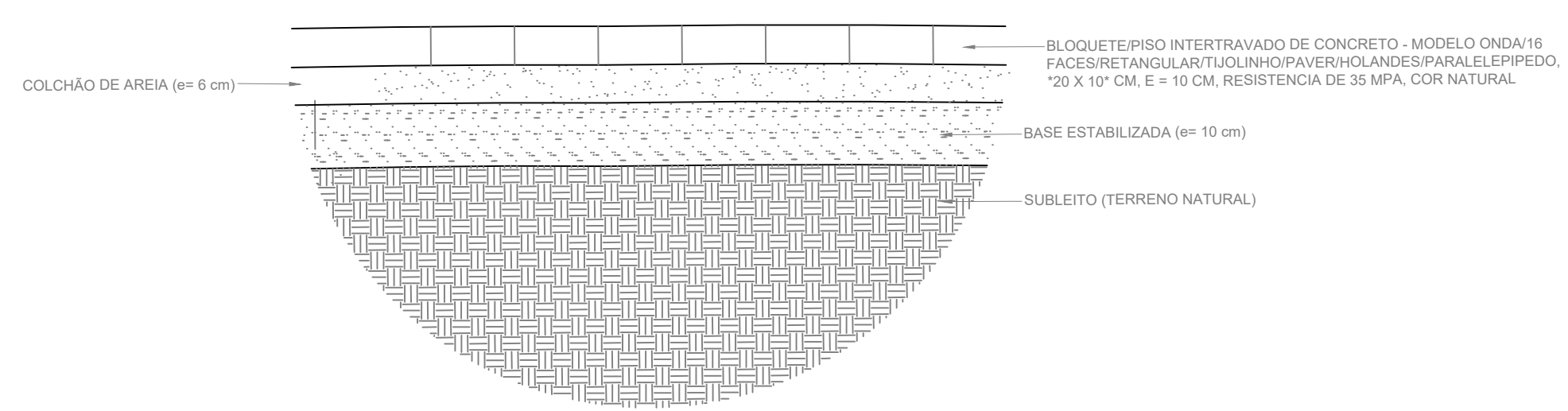
DETALHE PISO INTERTRAVADO
