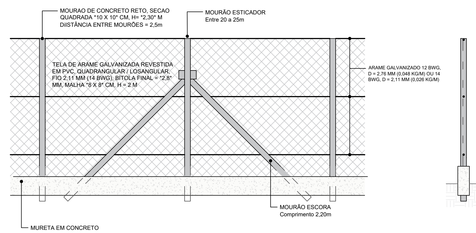
DETALHE CERCAMENTO
