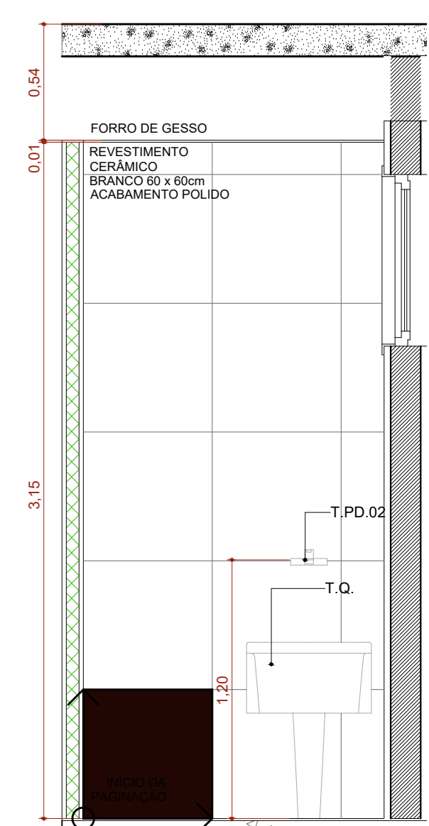
A.M.04 VISTA 04 Escala: 1:25
