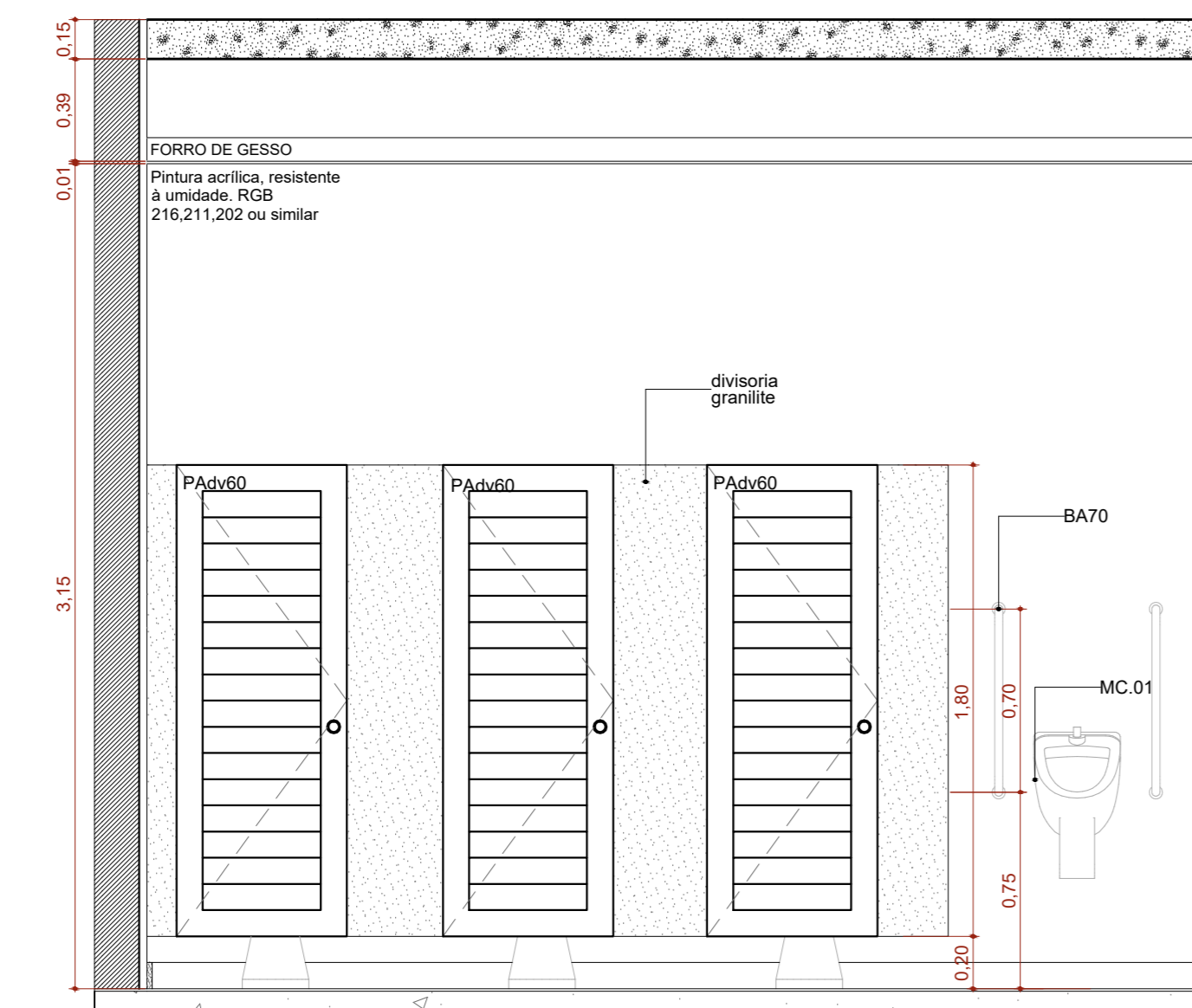
A.M.02 VISTA 01 Escala: 1:25
