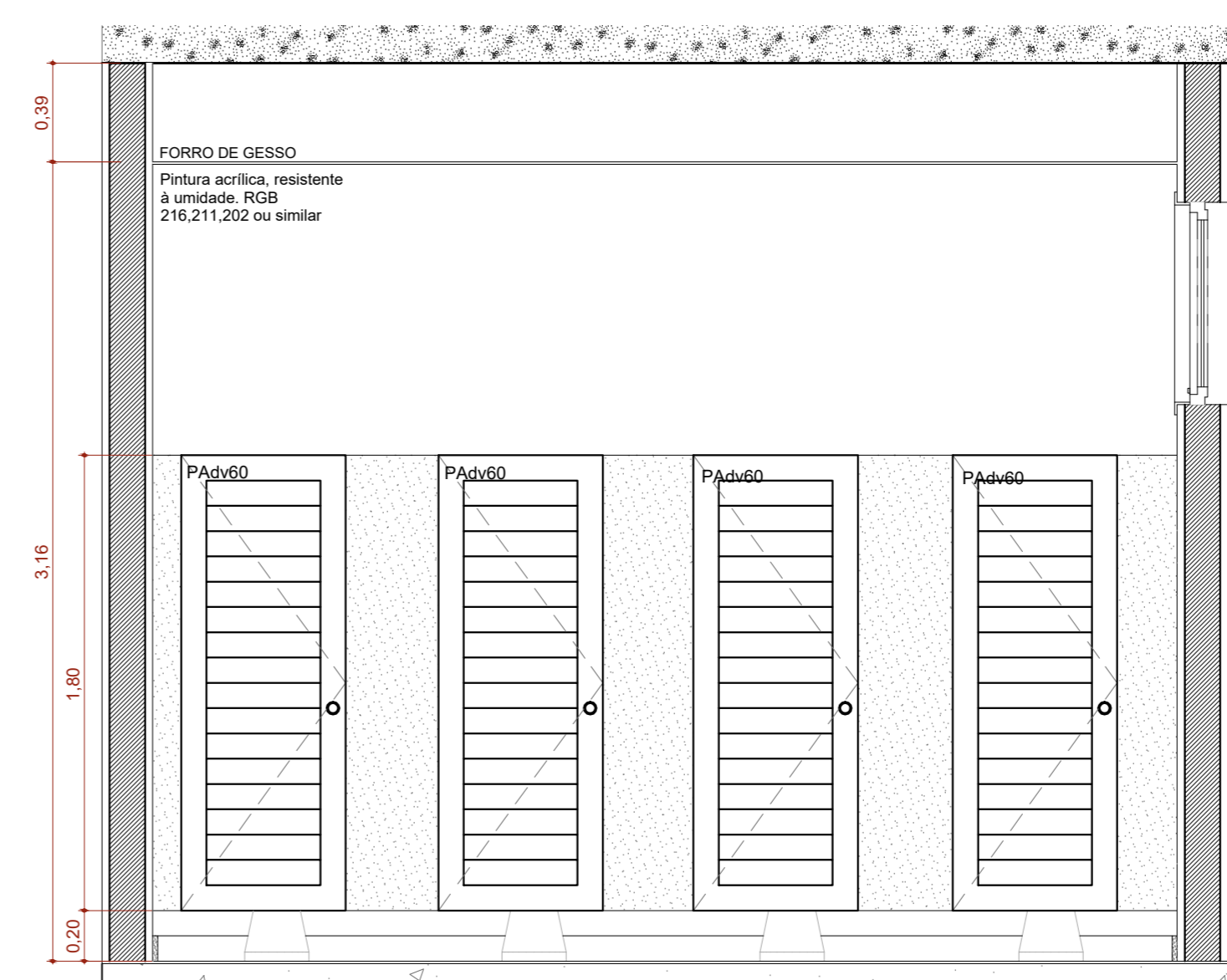
A.M.01 VISTA 04 Escala: 1:25
