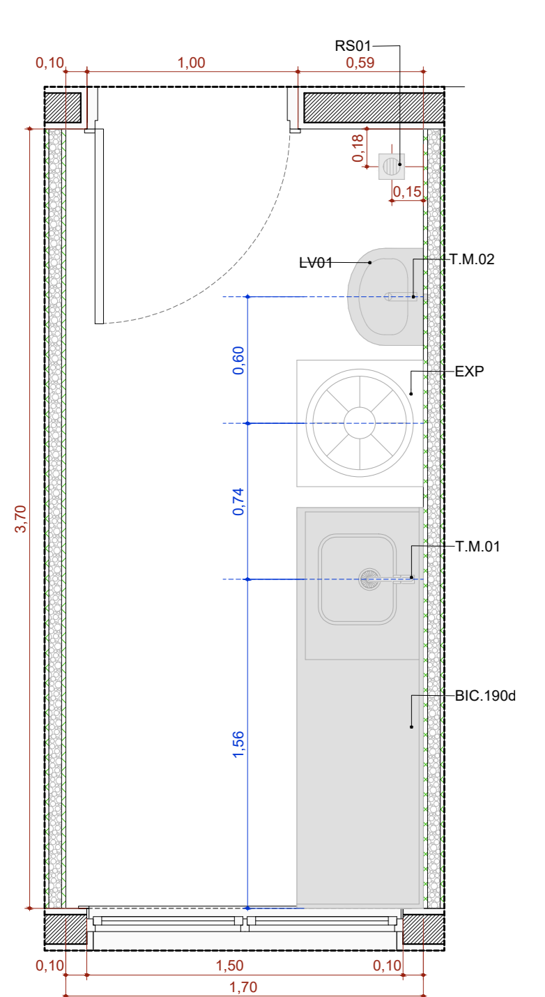
A.M.05 Utilidades Escala: 1:25
