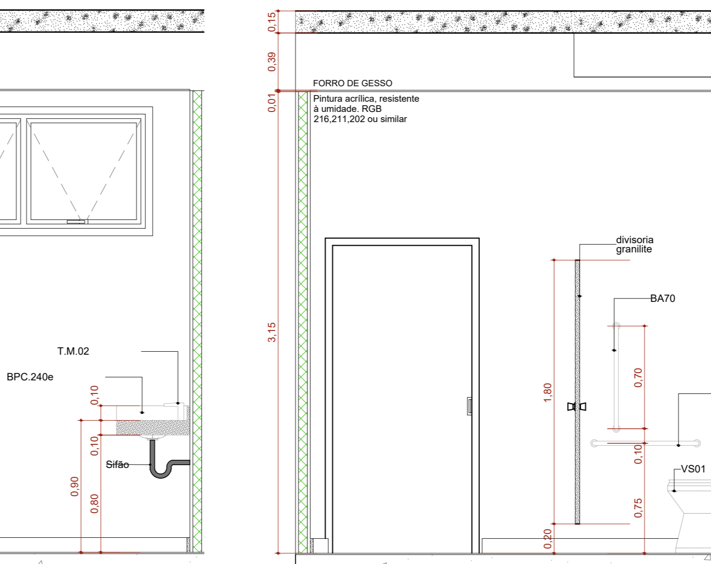
A.M.02 VISTA 04 Escala: 1:25
