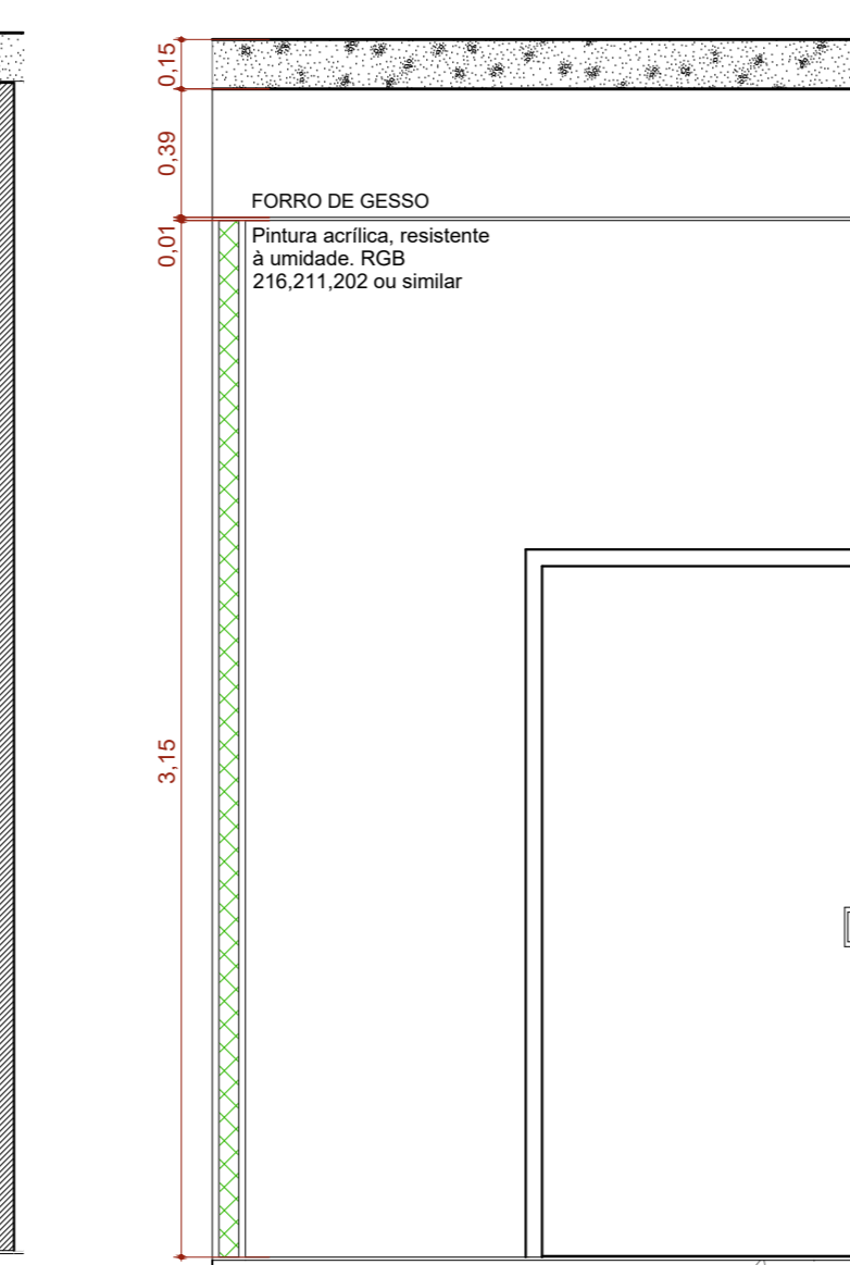
A.M.03 VISTA 03 Escala: 1:25
