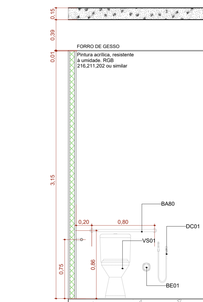
A.M.03 VISTA 02 Escala: 1:25
