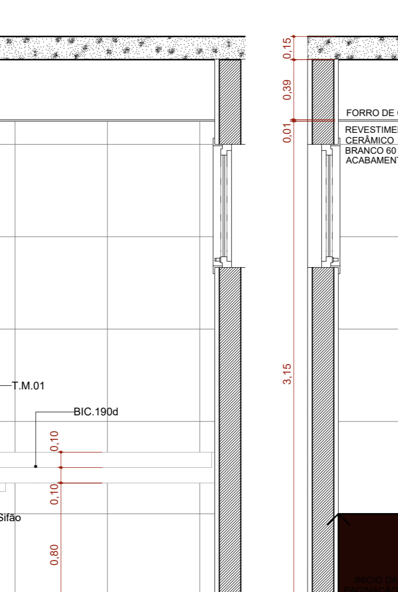
A.M.05 VISTA 03 Escala: 1:25
