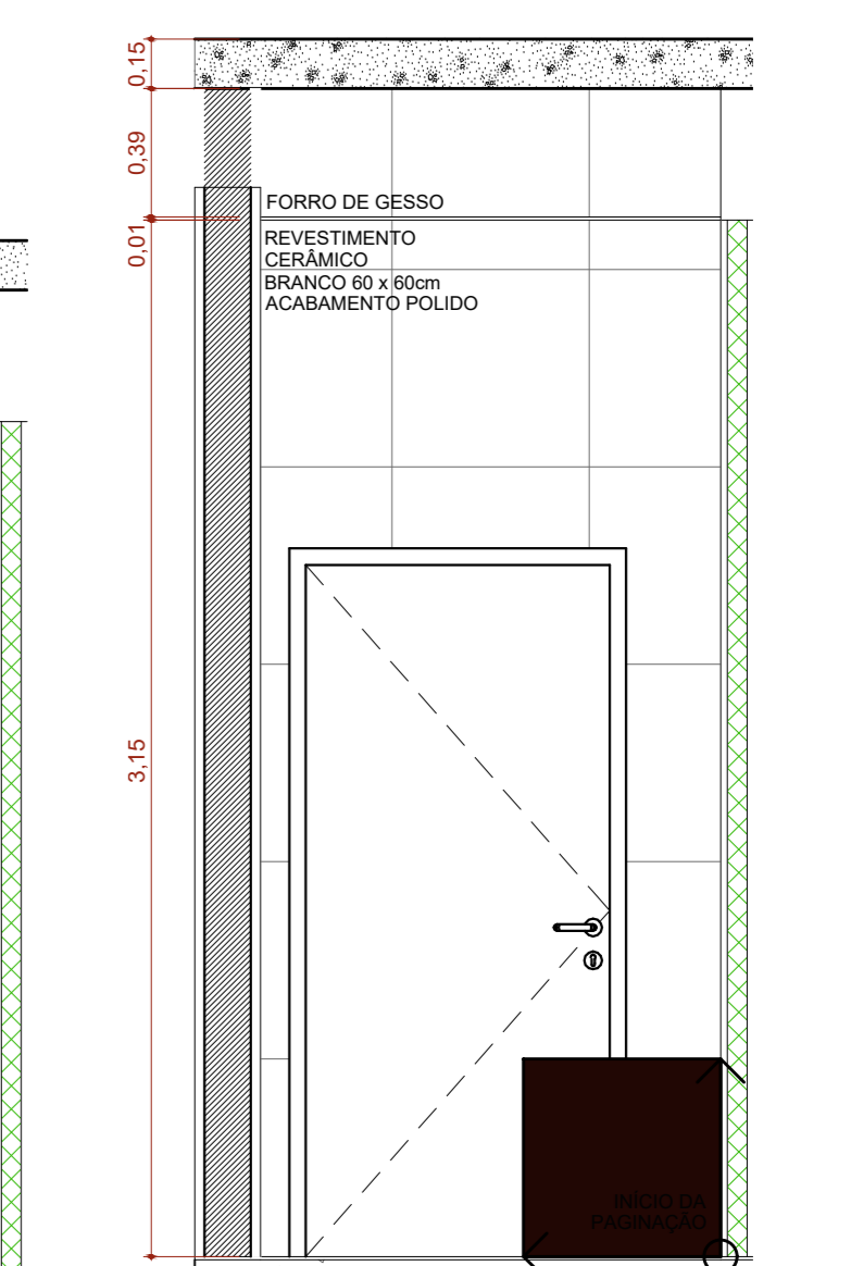
A.M.04 VISTA 03 Escala: 1:25
