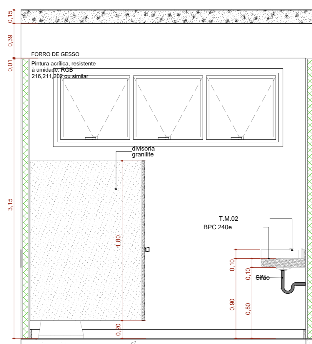
A.M.01 VISTA 02 Escala: 1:25
