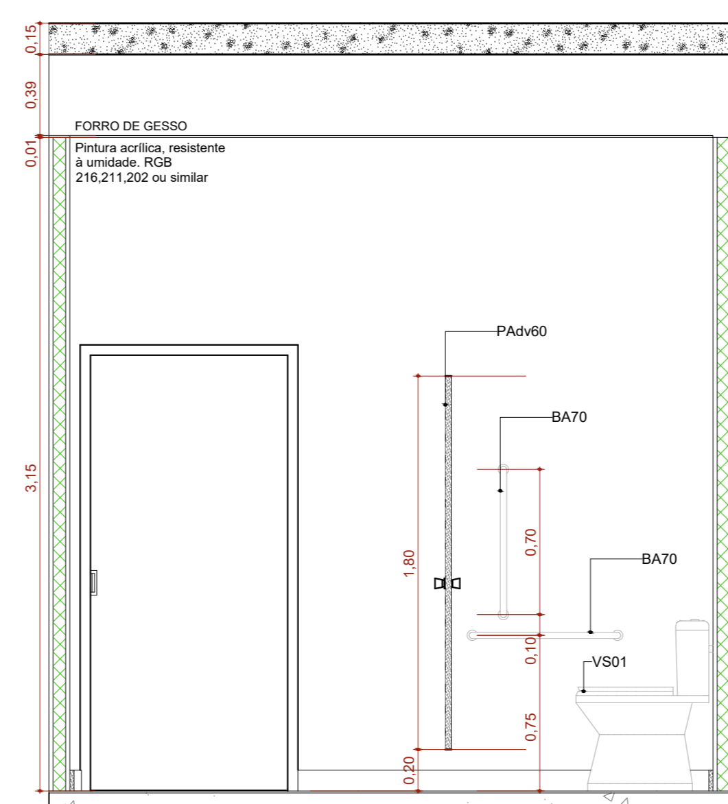
A.M.01 VISTA 03 Escala: 1:25
