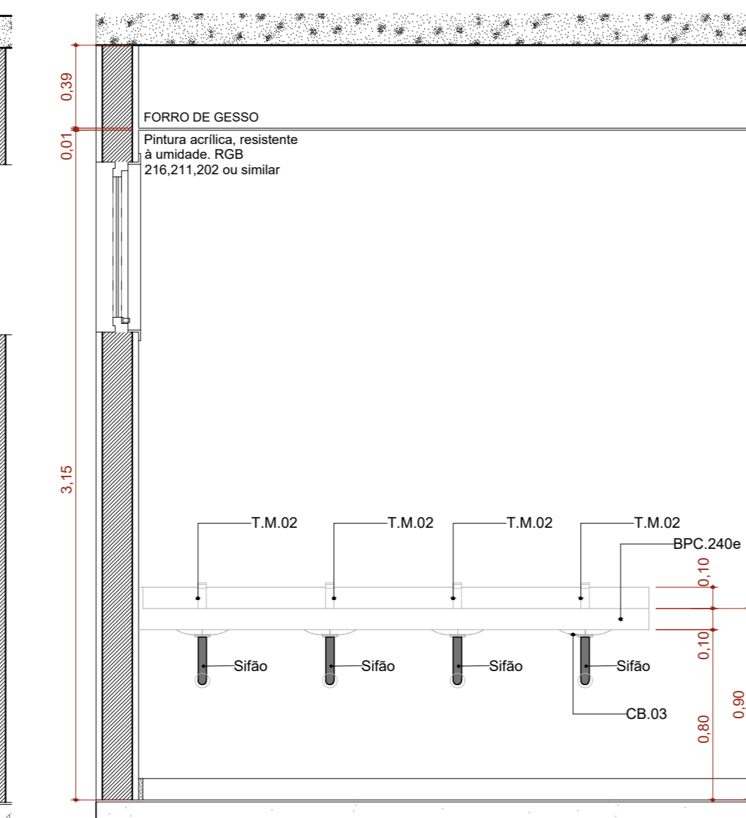
A.M.02 VISTA 02 Escala: 1:25
