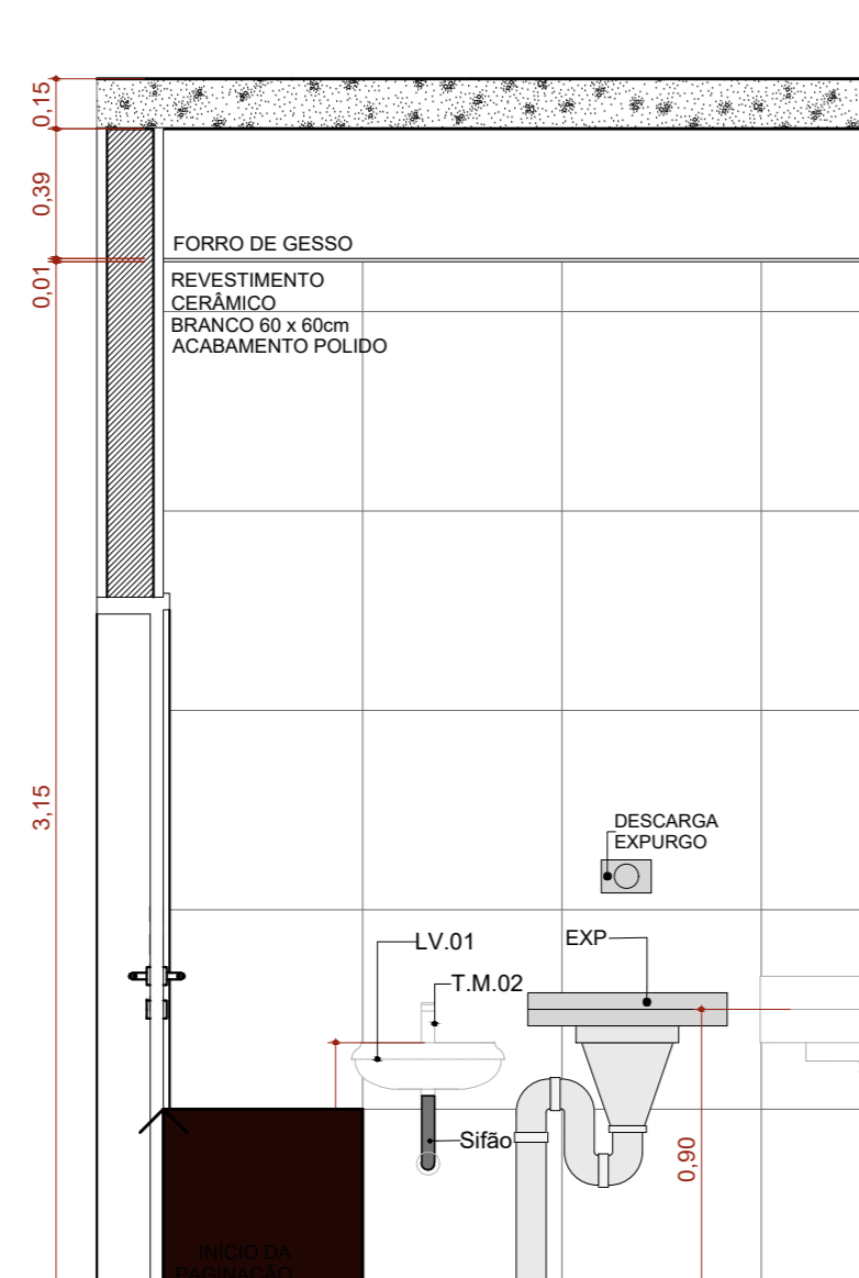
A.M.05 VISTA 02 Escala: 1:25
