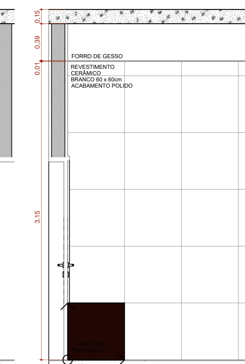
A.M.04 VISTA 02 Escala: 1:25
