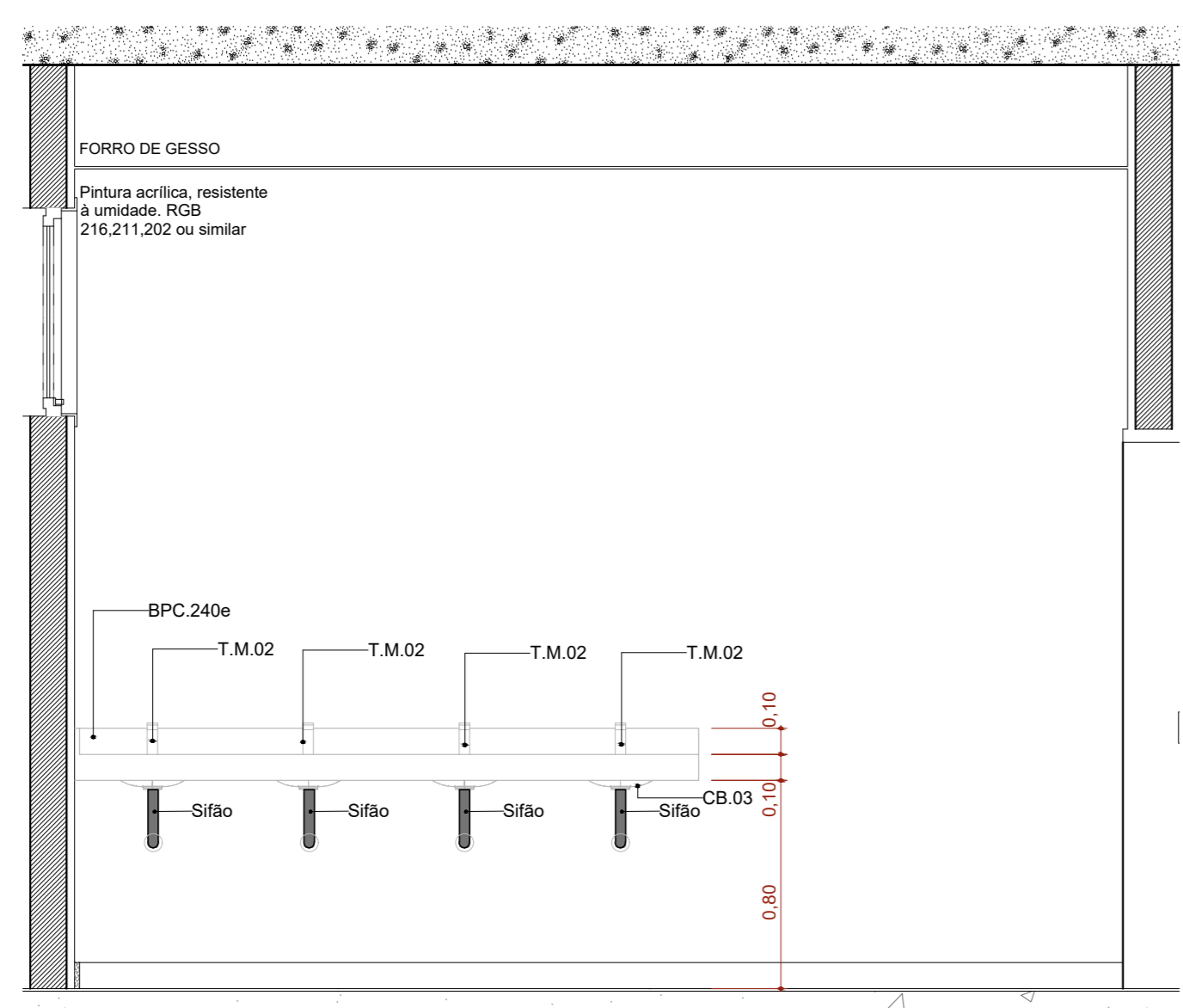
A.M.01 VISTA 01 Escala: 1:25
