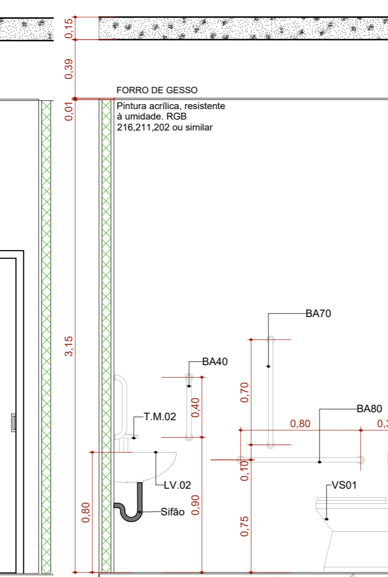
A.M.03 VISTA 04 Escala: 1:25
