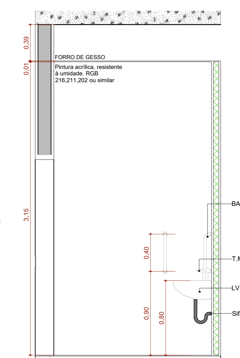
A.M.03 VISTA 01 Escala: 1:25
