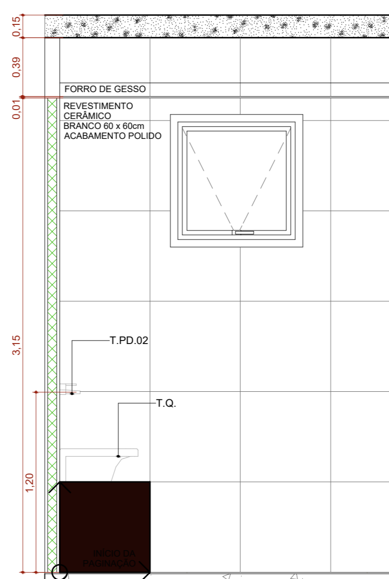
A.M.04 VISTA 01 Escala: 1:25
