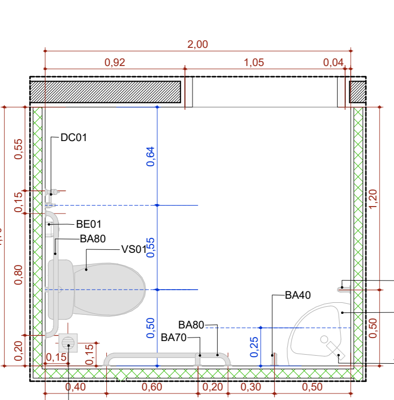
A.M.03 Sanit. PCD Escala: 1:25
